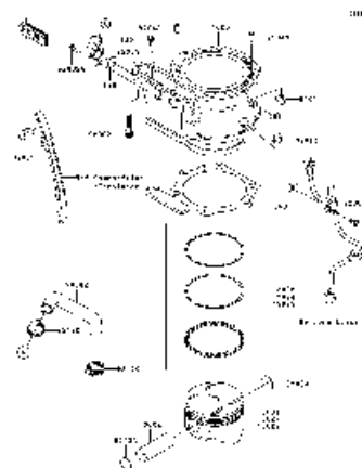
B-5 Cylinder/Piston(s)
