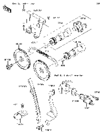
B-10 Camshaft(s)/Tensioner
