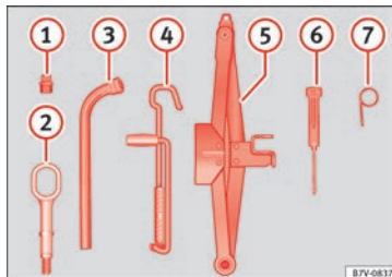
Fig. 63 En el maletero, bajo la cubierta de la superficie de carga: herramientas de a bordo.
