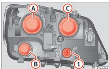
Fig. 104 En el vano motor: revestimientos en el faro izquierdo. A luces de cruce, B luz diurna y C luz de carretera y luz de posición.
