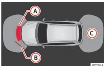
Fig. 209 Indicación del OPS en pantalla: (A) se ha detectado un obstáculo en la zona de colisión; (B) se ha detectado un obstáculo en el segmento; (C) zona registrada detrás del vehículo.
