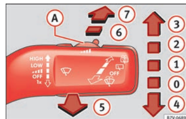
Fig. 43 Manejo del limpiaparabrisas y limpiapluneta.
