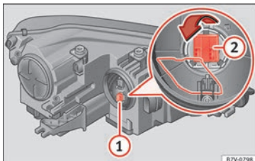
Fig. 107 Portalámparas del intermitente (1) y luz para curvas (2).
