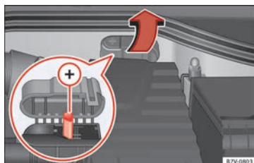
Fig. 73 En el vano motor: polo positivo de ayuda de arranque (+).
