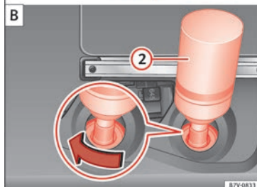
Fig. 238 Depósito de AdBlue con cierre de la boca de llenado y botella para reponer.
