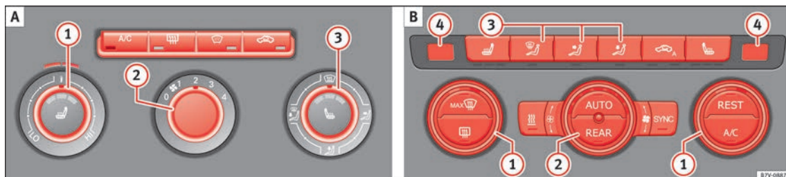
Fig. 51 Detalle de la consola central: A Mandos del Aire acondicionado manual eléctrico; B Mandos del Climatronic.
