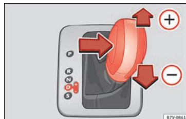
Fig. 202 Palanca selectora en la posición Tiptronic (vehículos con volante a la izquierda). Los vehículos con el volante a la derecha están dispuestos de forma simétrica.
