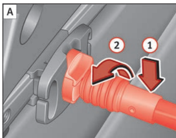
Fig. 170 Desenganche la red para el equipaje.
