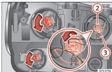
Fig. 105 Faro izquierdo.
