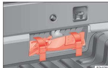
Fig. 98 En el maletero, visto desde el interior del vehículo: herramientas de a bordo en una cavidad situada en la zona del portacierres.
