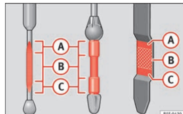
Fig. 53 Varilla de medición del nivel de aceite.
