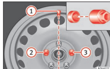
Fig. 67 Cambio de rueda: válvula del neumático ① y ubicación del tornillo antirrobo de la rueda ② o ③.
