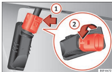
Fig. 115 Luz de la matrícula: Desmontar el portalámparas.
