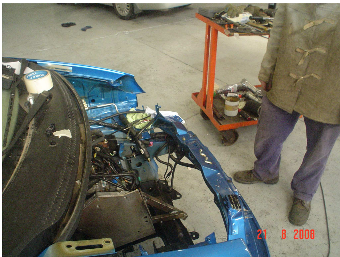
Se diseña la platina de acople del motor eléctrico con la caja de cambios. En hierro de 7 mm de espesor.
