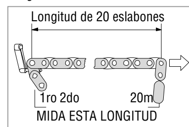
Longitud cadena de transmisión
