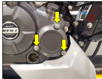
Perno de la tapa del filtro de aceite
