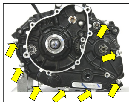
Pernos de la unión del cárter
