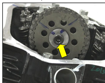
Perno allen del piñón de levas
