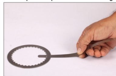
Alabeo plato separador del embrague
