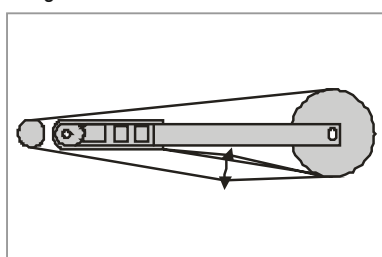
Holgura de la cadena de transmisión
