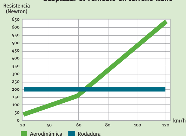
Resistencias que ha de vencer el motor para desplazar el vehículo en terreno llano
