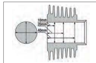
Diámetro interno del cilindro
