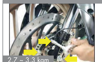
Tornillos disco delantero
