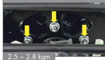
Tuercas sprocket trasero
