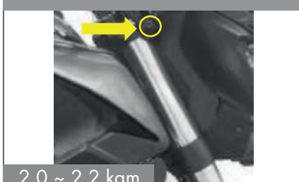
Tornillos de horquilla inferior
