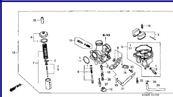
M-17 Carburador / Carburetor / Carburador
