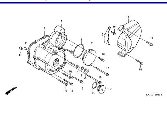
M-8 Tampa Lateral Esquerda / Left Crankcase Cover / Cubierta Izquierda del Cáster Motor
