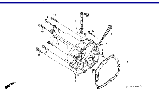
M-8 Tampa Lateral Esquerda / Left Crankcase Cover / Cubierta Izquierda del Cáster Motor
