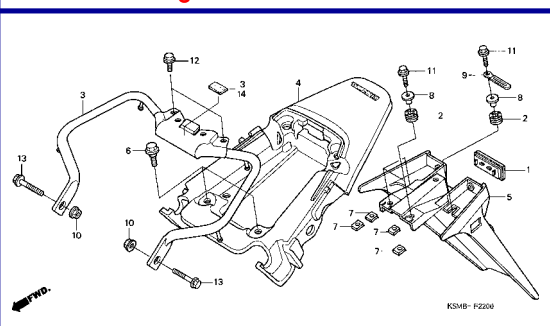
C-22 Pára-Lama Traseiro / Rear Fender / Parafango Trasero
