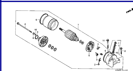
M-11 Motor de Partida / Starting Motor / Motor Arranque
