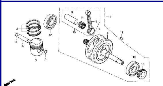
M-13 Árvore de Manivelas • Pistão / Crankshaft • Pistón / Cigüeñal • Pistón
