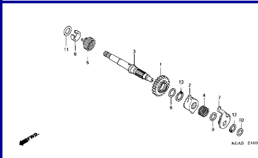
M-16 Sistema de Partida / Kick Starter Spindle / Arranque de Pie
