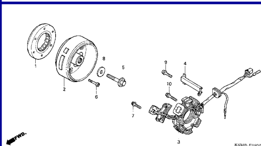
M-9 Gerador / Generator / Generador
