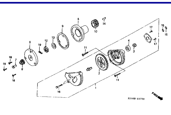
M-7 Bomba de Óleo / Oil Pump / Bomba de Aceite
