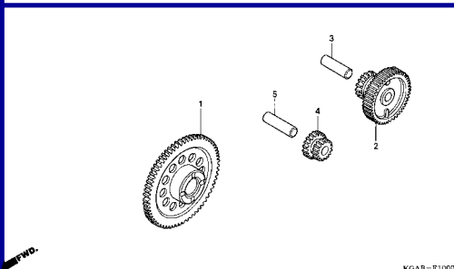
M-10 Embreagem Partida / Starting Clutch / Embrague Arranque
