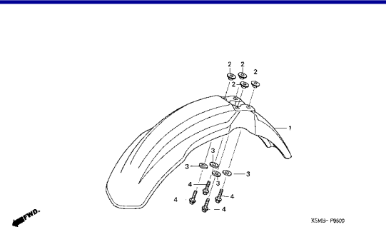
C-6 Pára-Lama Dianteiro / Front Fender / Parafango Delantero
