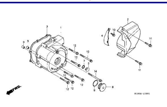
M-8.1 Tampa Lateral Esquerda / Left Crankcase Cover / Cubierta Izquierda del Cáster Motor
