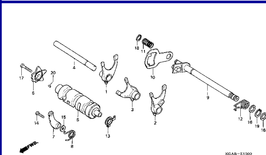
M-15 Tambor Seletor / Gearshift Drum / Tambor de Cambio
