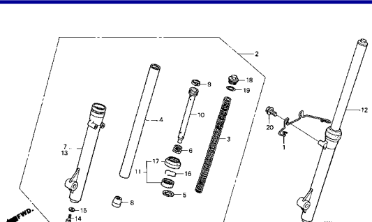
C-7 Garfo Dianteiro / Front Fork / Horquilla Delantera
