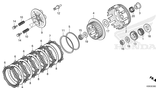
CLUTCH
