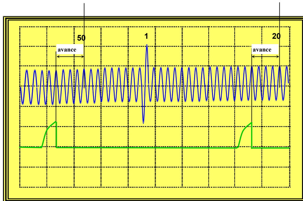
PMS Cilindros 2-3
