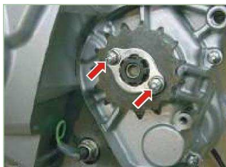
Tornillos seguro sprocket salida 1.1 Kg.-m
