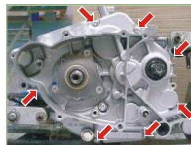
Tornillos de carter 1.1 Kg.-m
