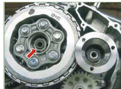
Tuerca clutch (rosca izquierda) 4.5 Kg.-m
