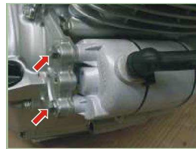
Tornillos marcha 1.1 Kg.-m
