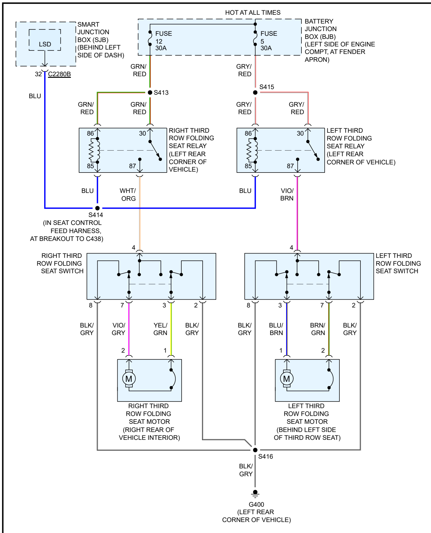
CIRCUITO DE ASIENTOS PLEGABLES DE LA TERCERA FILA
