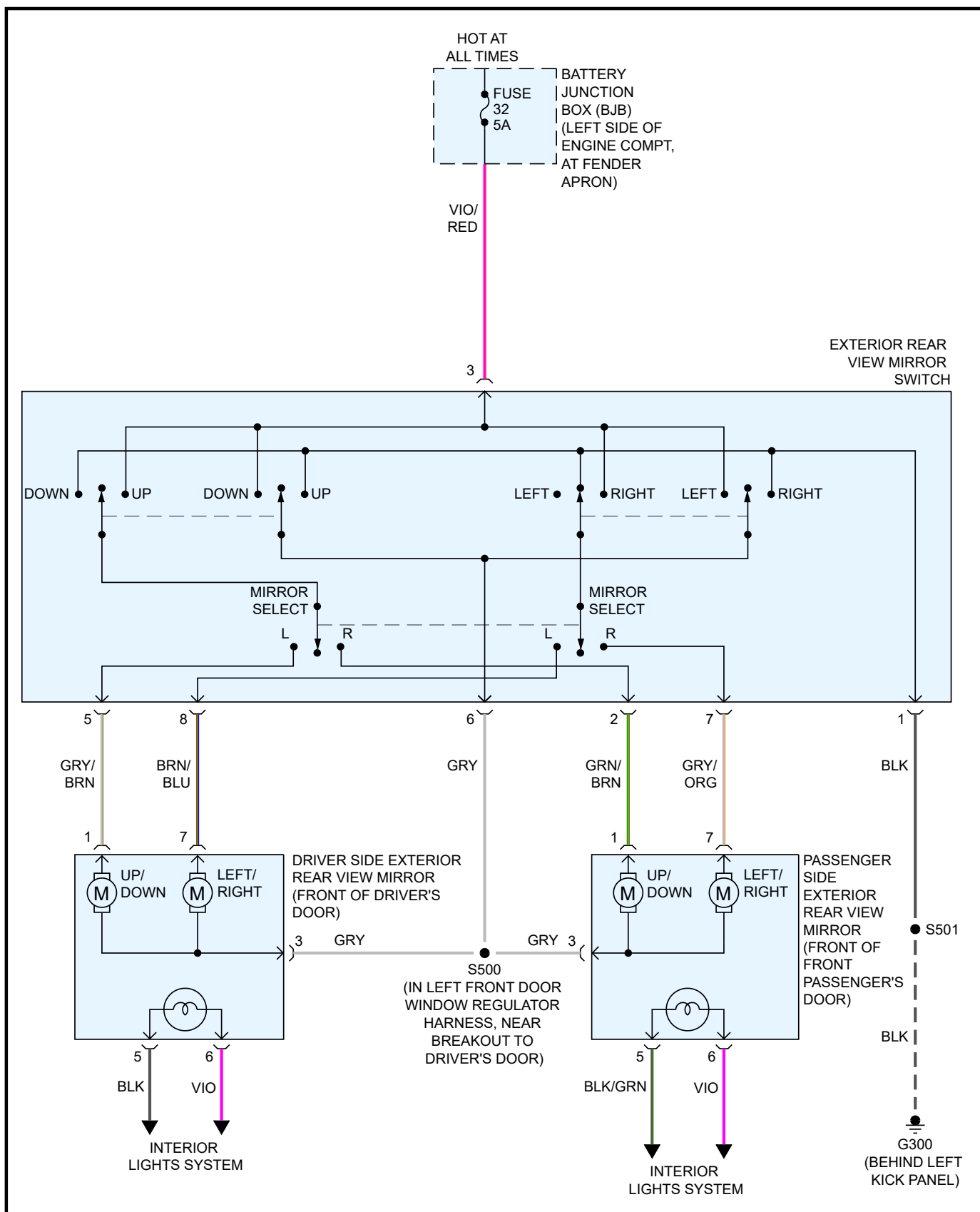
CIRCUITO DE ESPEJOS ELÉCTRICOS (SIN ESPEJOS TÉRMICOS)
