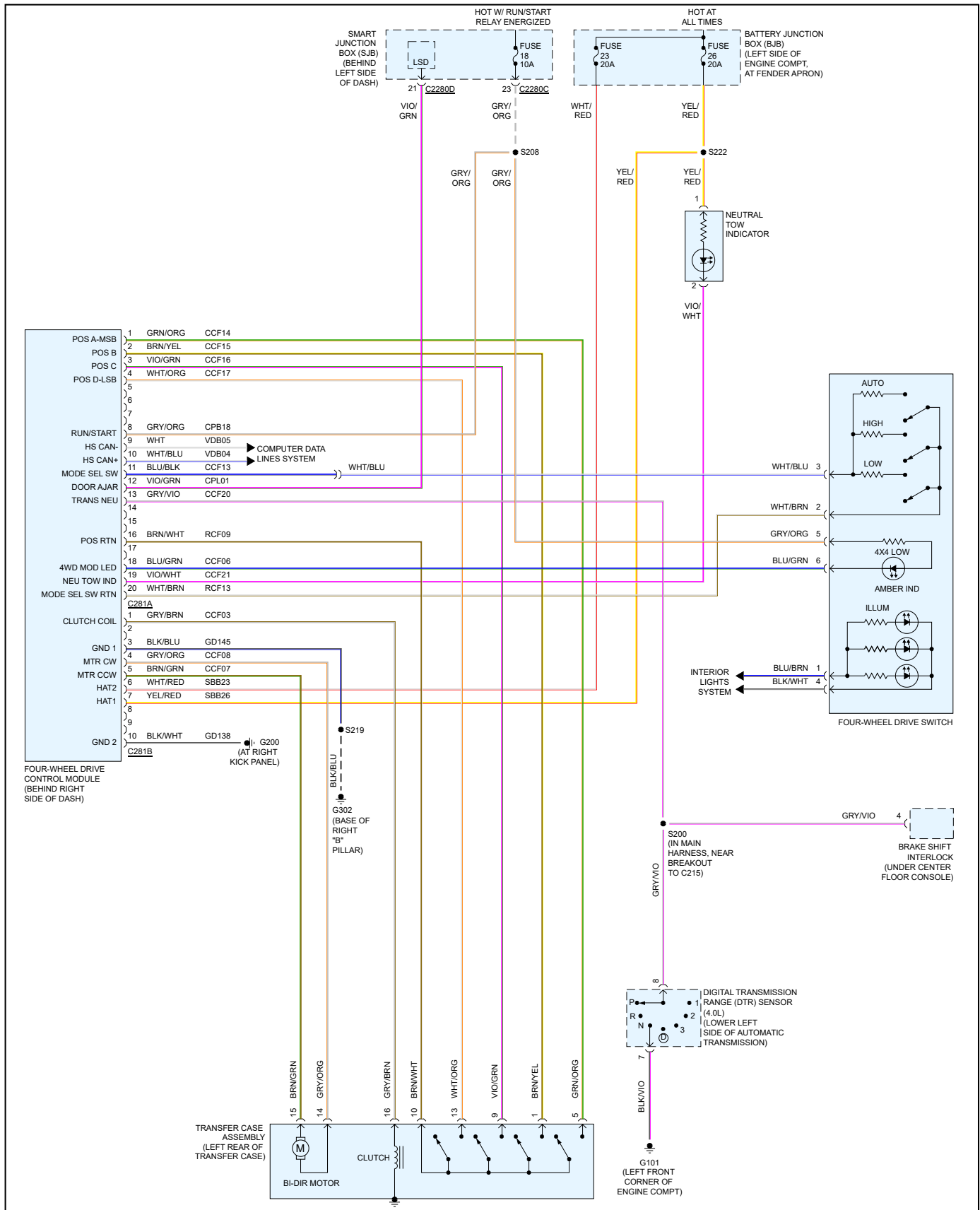
MODULO DE CONTROL DE LA TRANSMISION (TCM) 4WD
