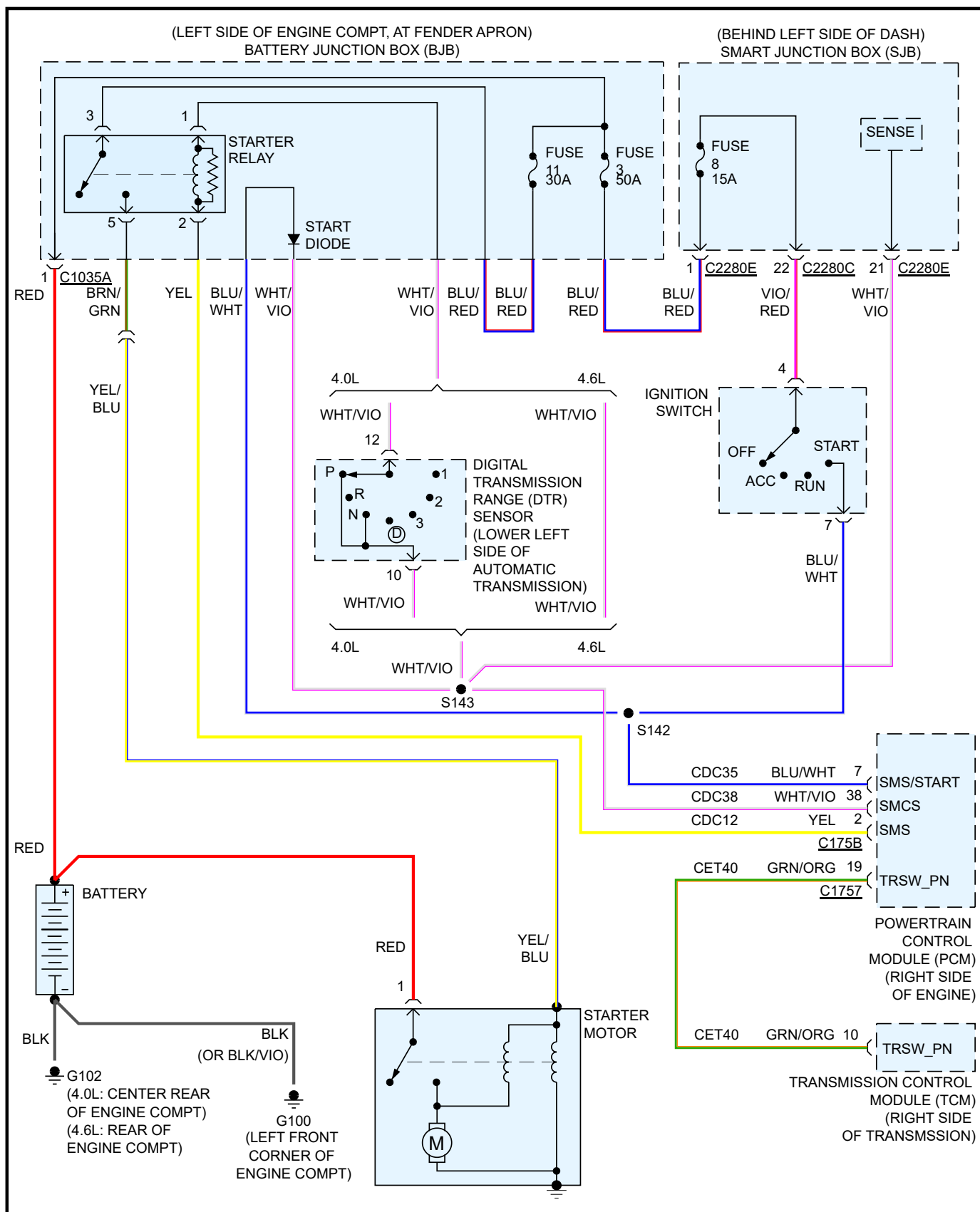
CIRCUITO DE ARRANQUE
