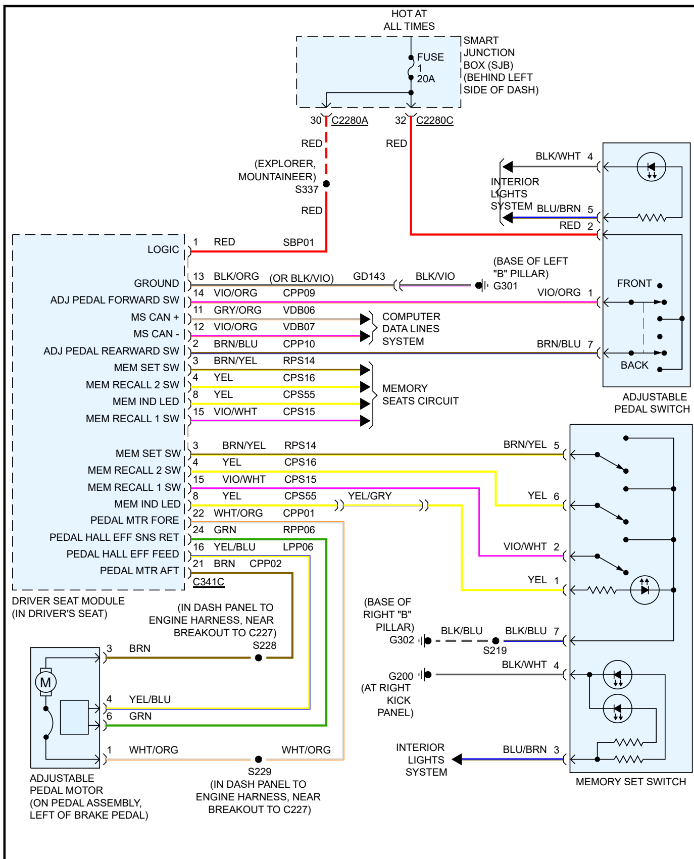
CIRCUITO DE PEDAL AJUSTABLE
