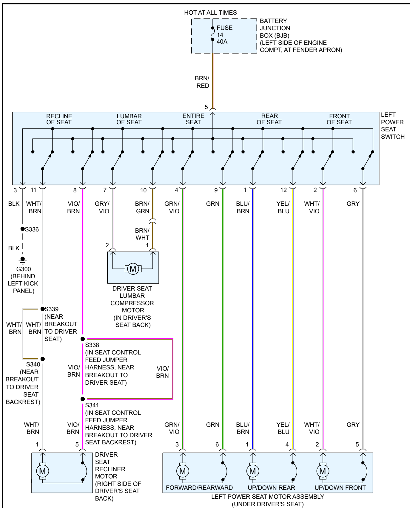
CIRCUITO DEL ASIENTO ELÉCTRICO DEL CONDUCTOR (CON ASIENTO ELÉCTRICO DE 10 POSICIONES)
