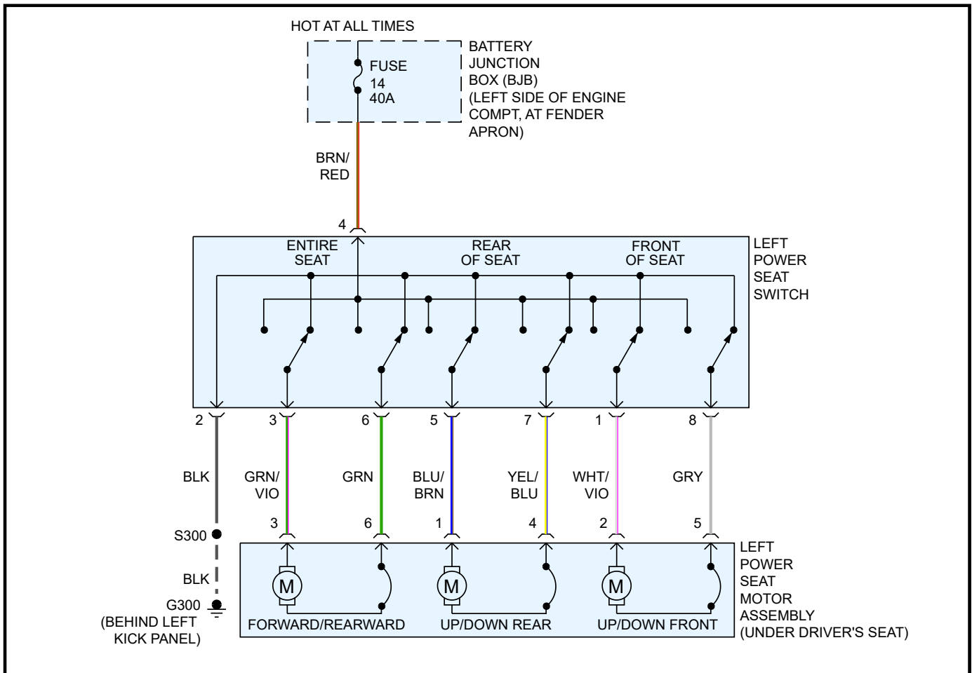
CIRCUITO DEL ASIENTO ELÉCTRICO DEL CONDUCTOR (CON ASIENTO ELÉCTRICO DE 6 POSICIONES)
