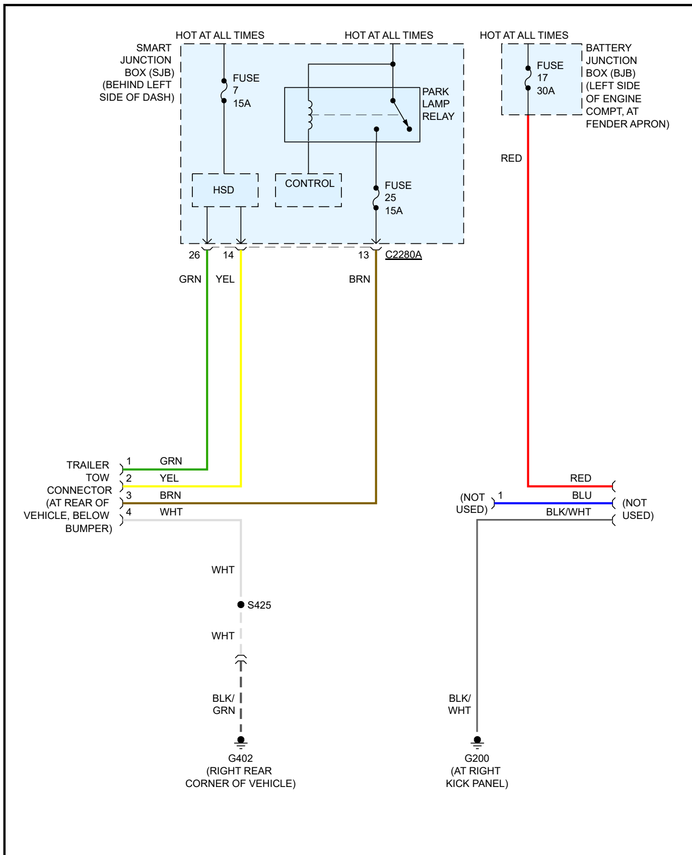
CIRCUITO DE REMOLQUE DE REMOLQUE (CON SERVICIO LIVIANO)
