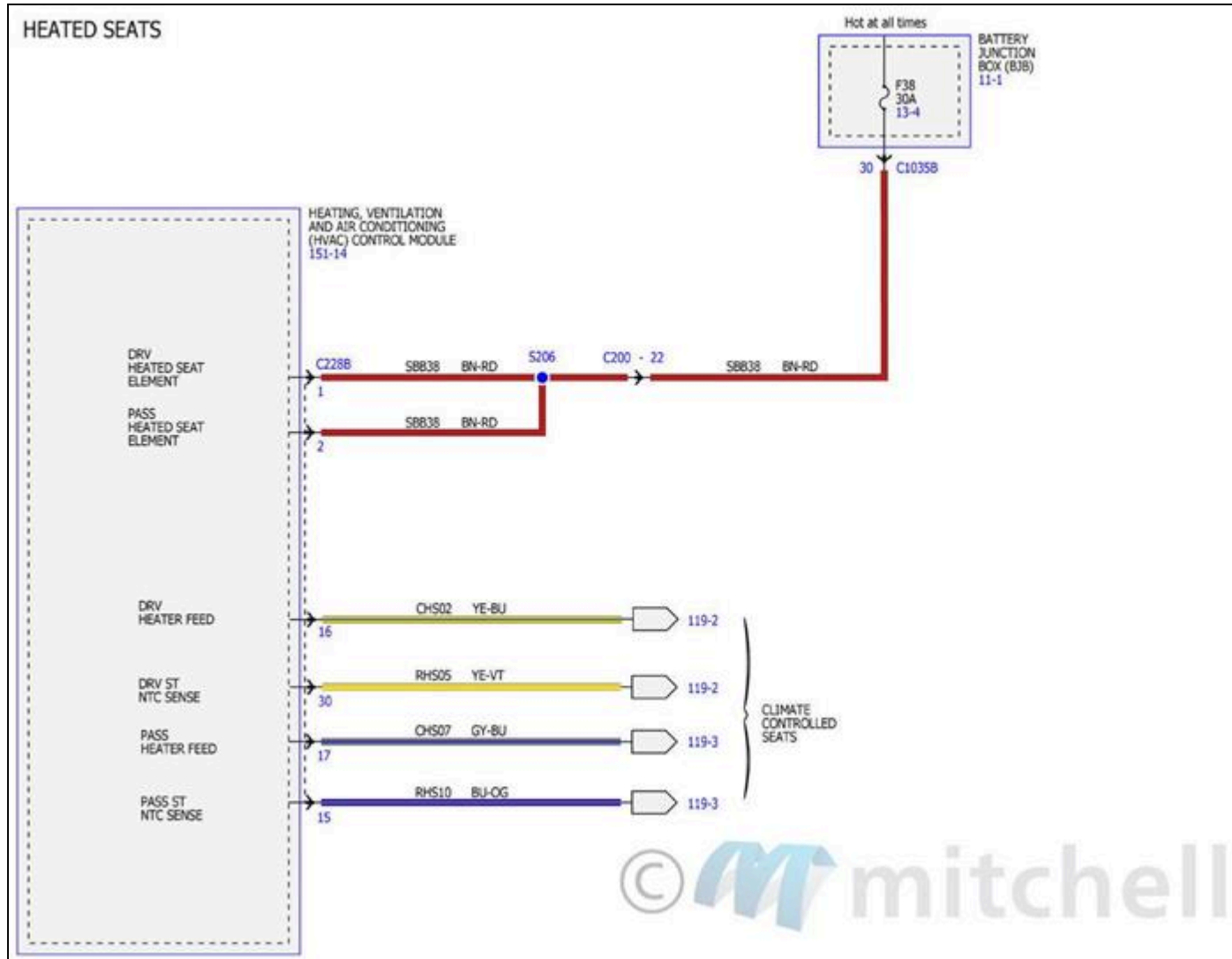
Fig. 20: Diagramas de cableado del sistema de control de clima automático (6 de 7)
