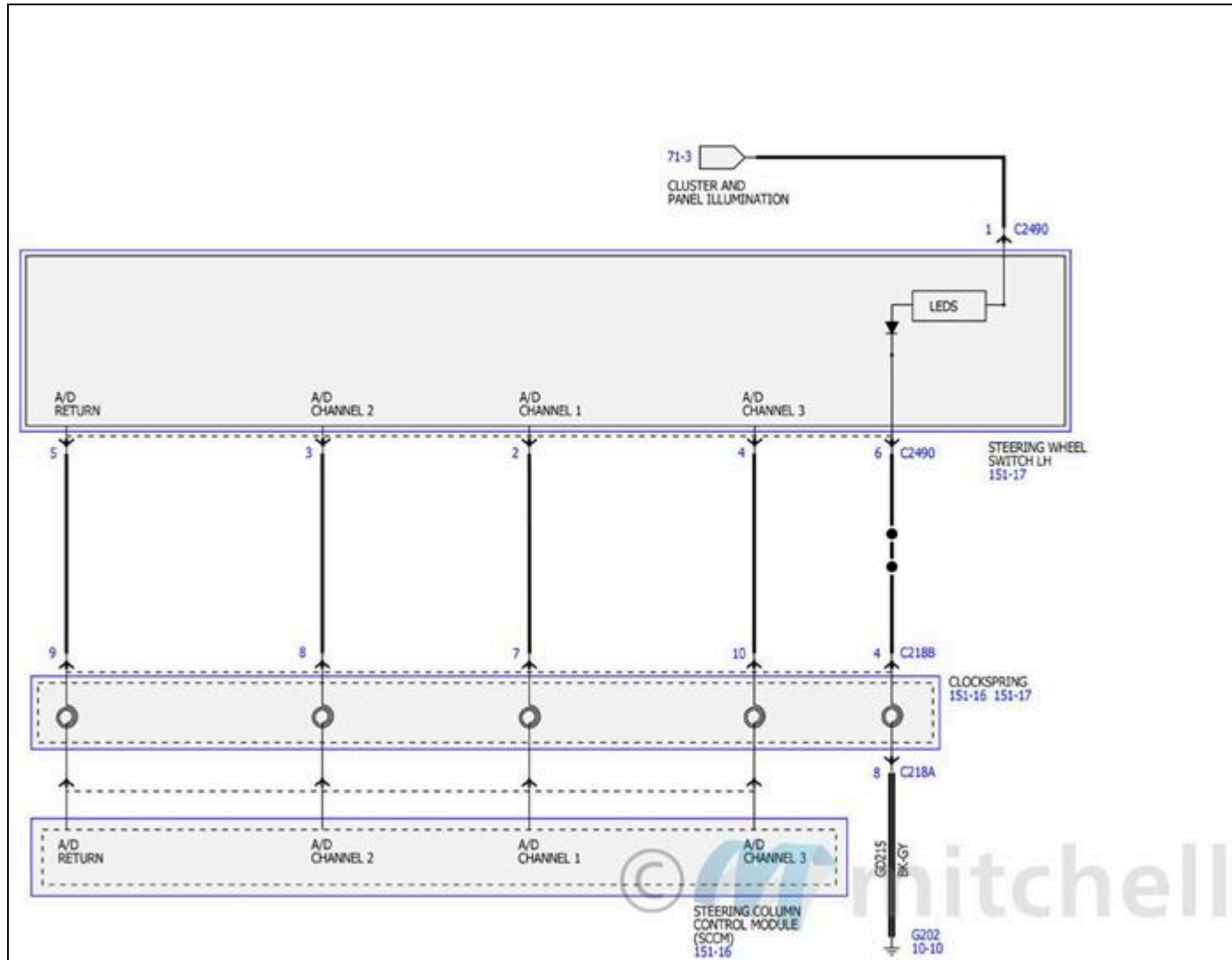
Fig. 36: Diagramas de cableado del control de cruceo (5 de 7)
