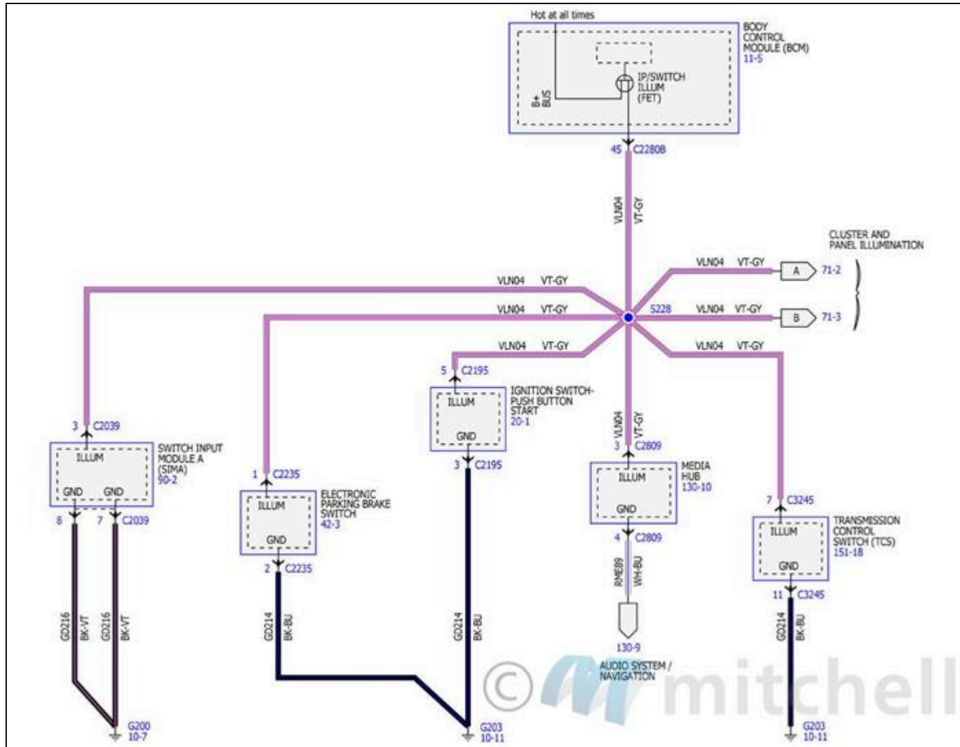
Fig. 27: Diagramas de cableado de iluminación de grupos y paneles (1 de 3)
