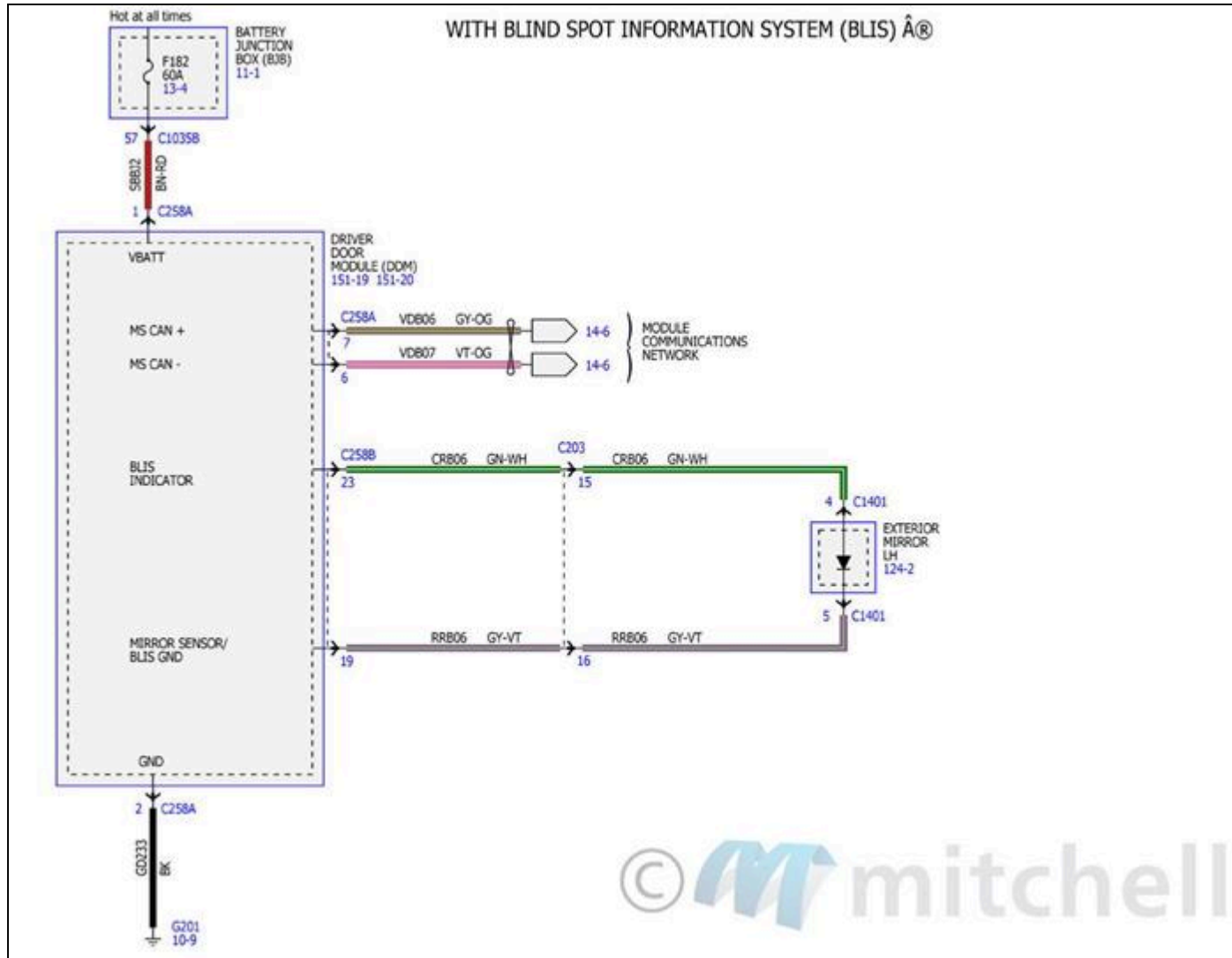
Fig. 220: Diagramas de cableado del sistema de mensajería de emergencia del vehículo (3 de 8)
