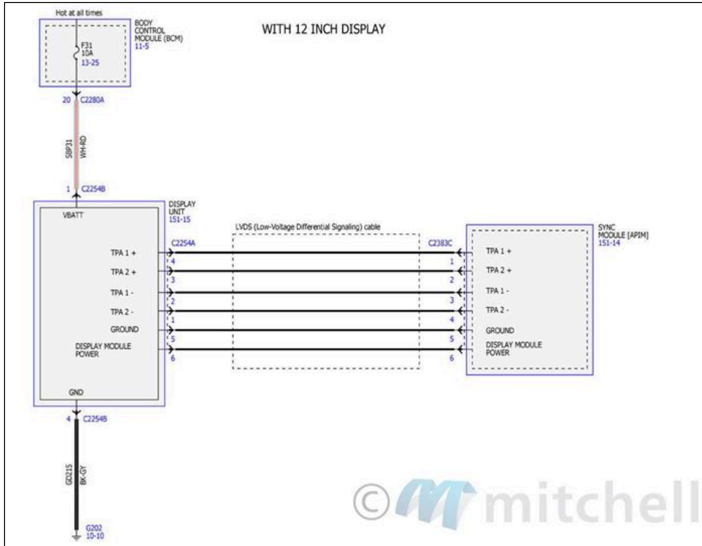
Fig. 3: Diagramas de cableado del sistema de audio (3 de 14)
