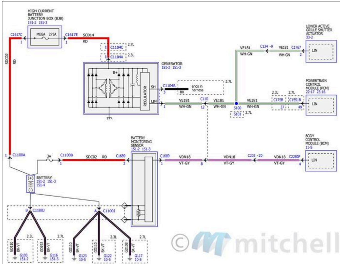
Fig. 22: Diagrama de cableado del sistema de carga
