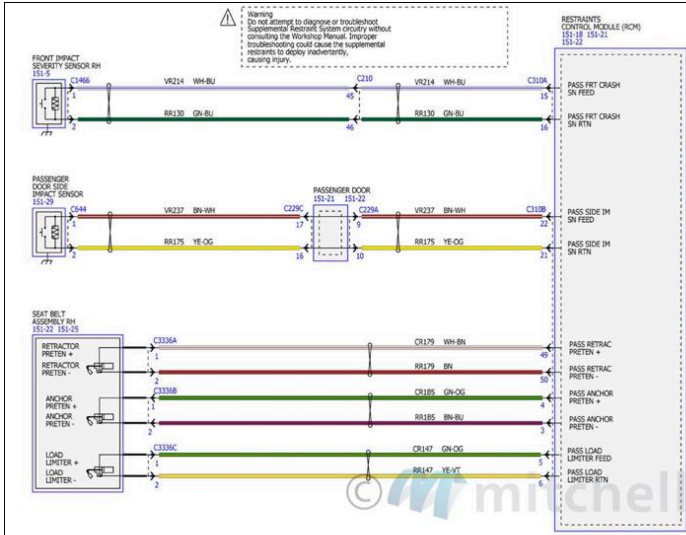
Fig. 192: Diagramas de cableado del sistema de retención suplementario (4 de 8)
