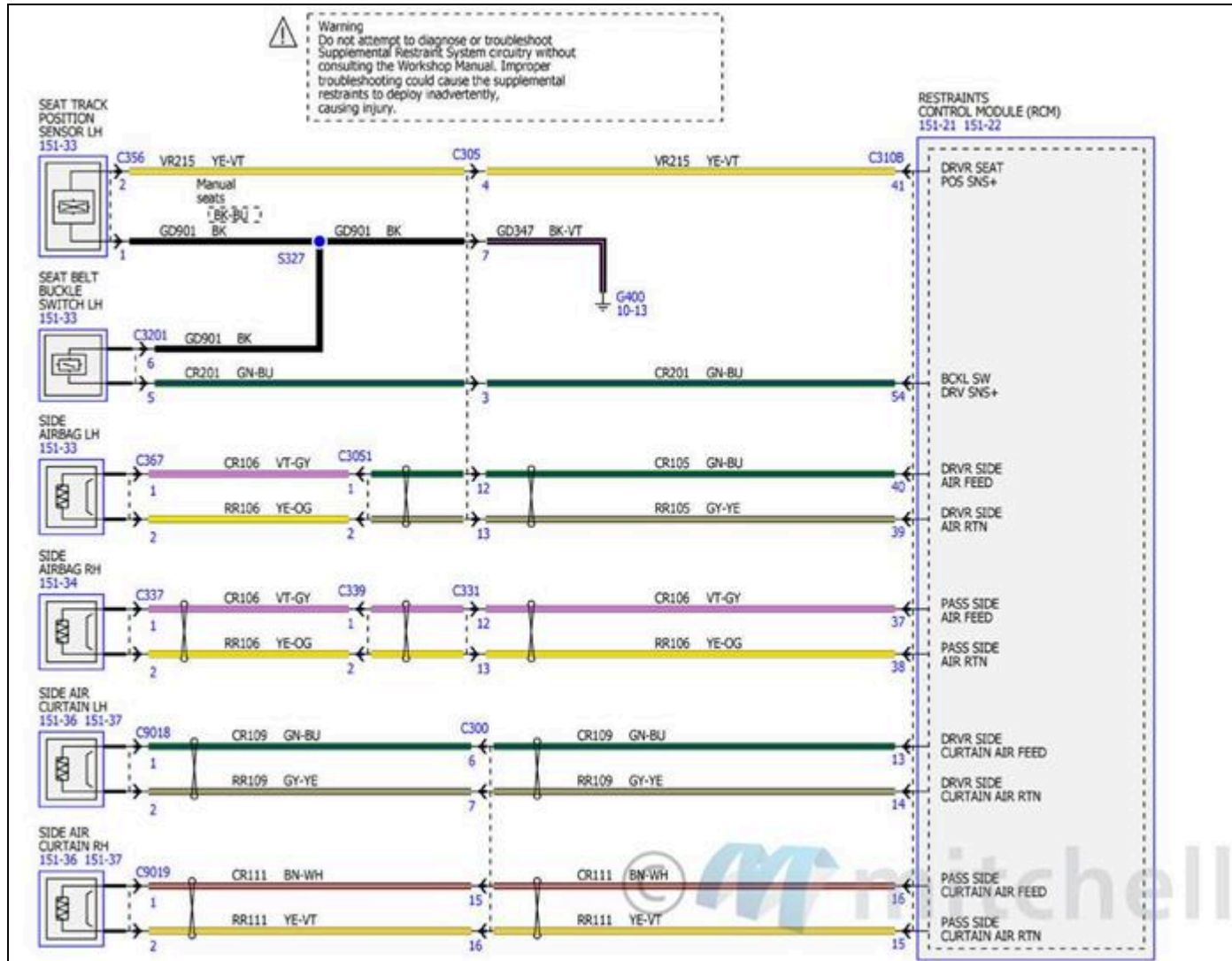
Fig. 194: Diagramas de cableado del sistema de retención suplementario (6 de 8)
