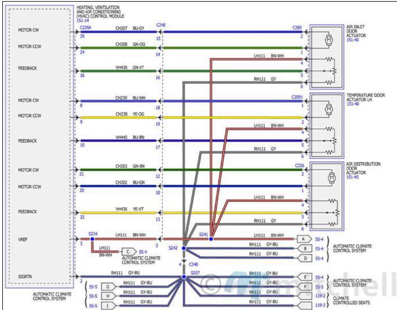
Fig. 17: Diagramas de cableado del sistema de control de clima automático (3 de 7)
