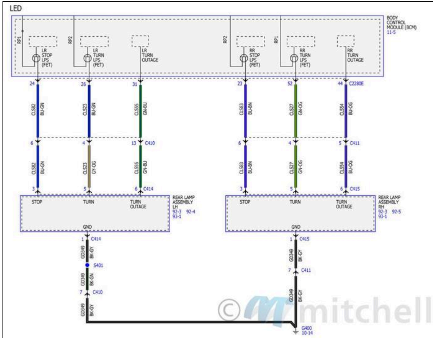
Fig. 211: Diagramas de cableado de luces de señal de giro, de freno y de emergencia (5 de 6)
