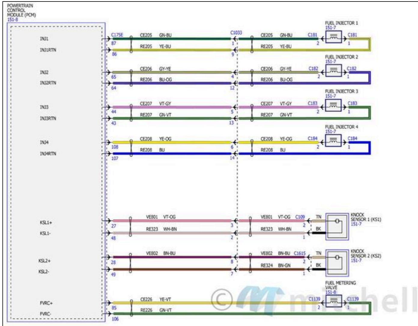
Fig. 45: Diagramas de cableado de los controles electrónicos del motor - 2.3L (3 de 17)
