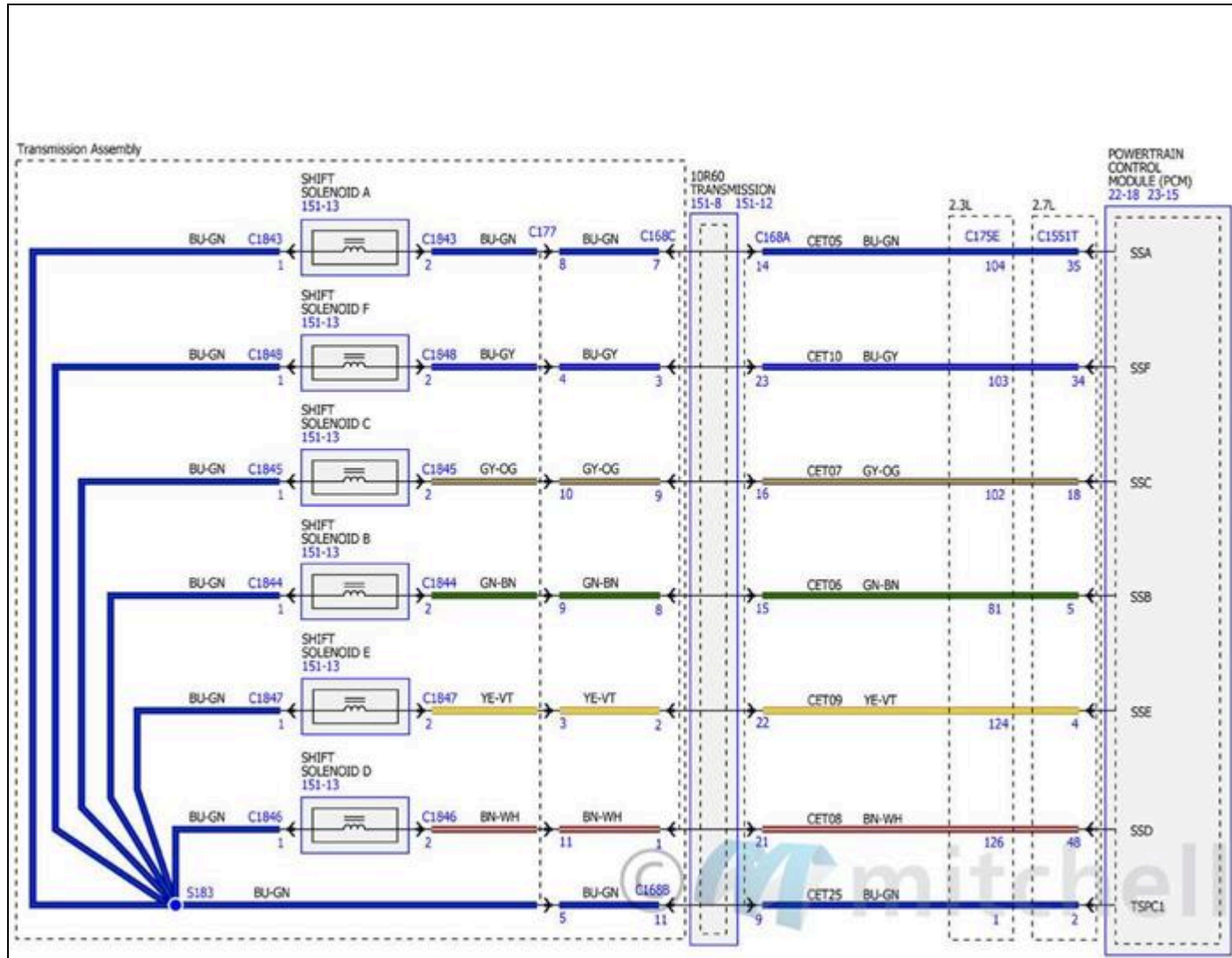
Fig. 204: Diagramas de cableado de los controles de transmisión - 10R60 (5 de 7)
