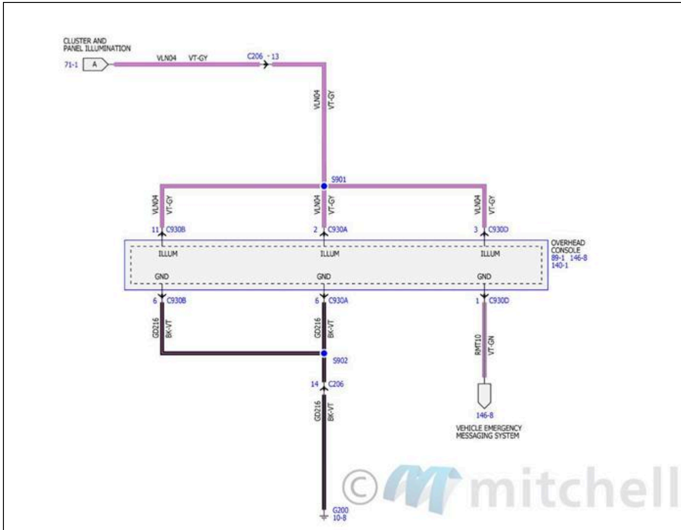
Fig. 28: Diagramas de cableado de iluminación de grupos y paneles (2 de 3)
