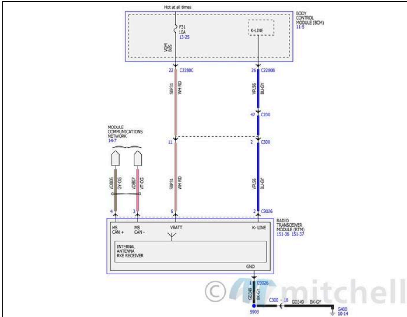
Fig. 197: Diagrama de cableado del sistema de control de presión de neumáticos
