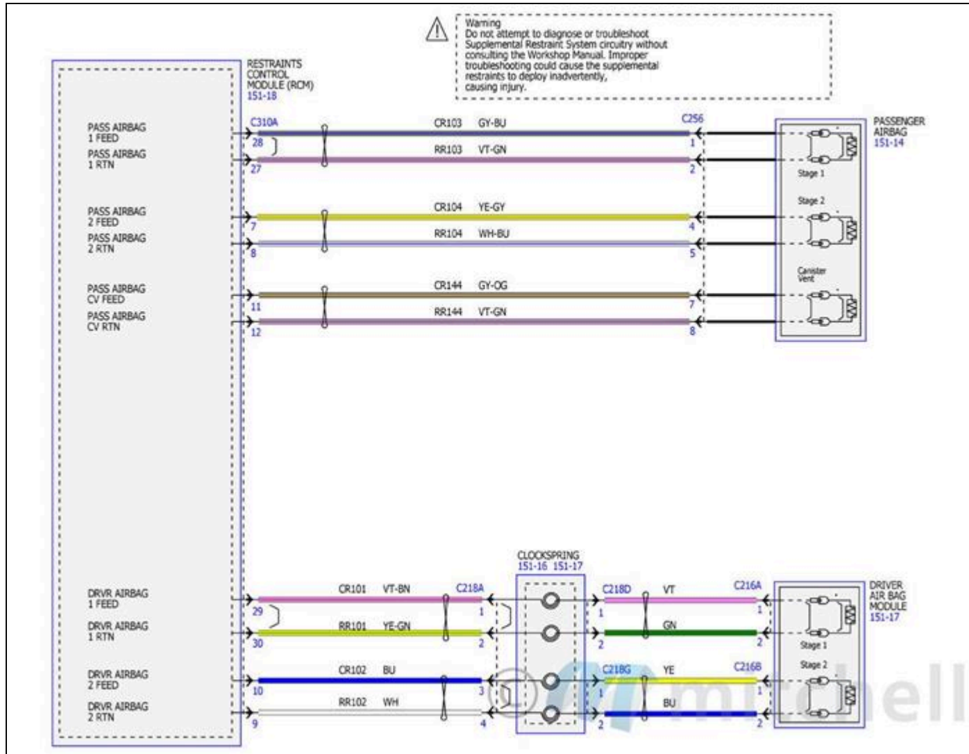
Fig. 196: Diagramas de cableado del sistema de retención suplementario (8 de 8)
