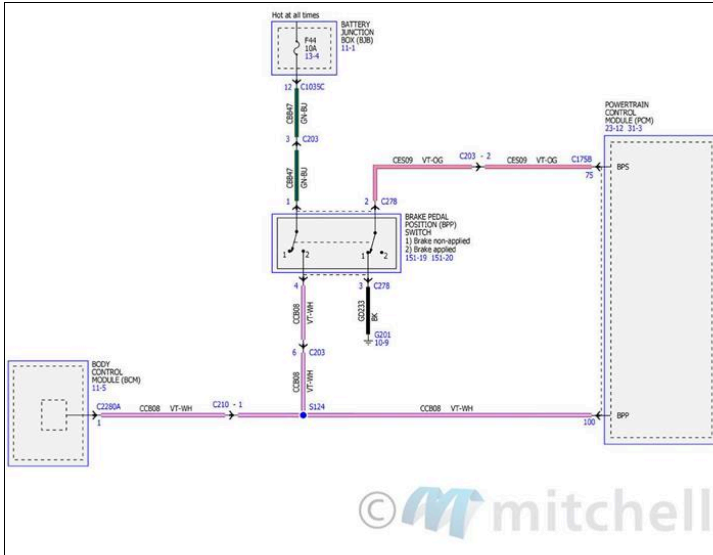
Fig. 212: Diagramas de cableado de luces de señal de giro, de freno y de emergencia (6 de 6)
