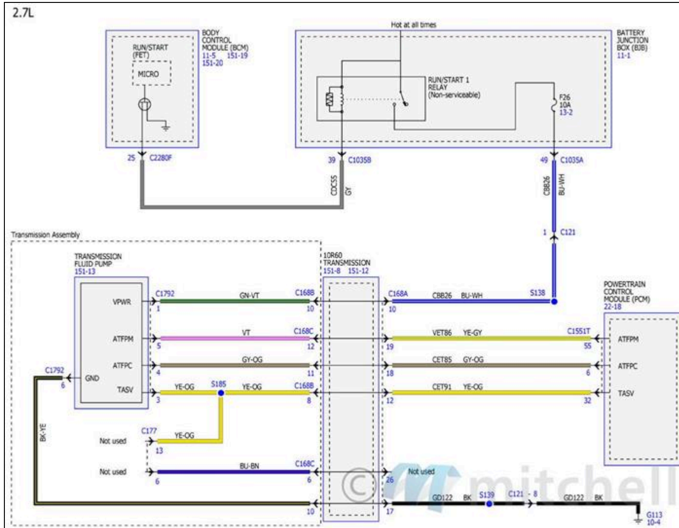
Fig. 200: Diagramas de cableado de los controles de transmisión - 10R60 (1 de 7)
