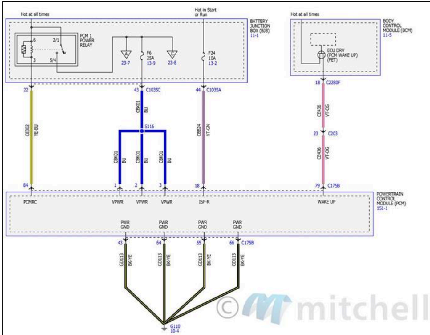
Fig. 43: Diagramas de cableado de los controles electrónicos del motor - 2.3L (1 de 17)
