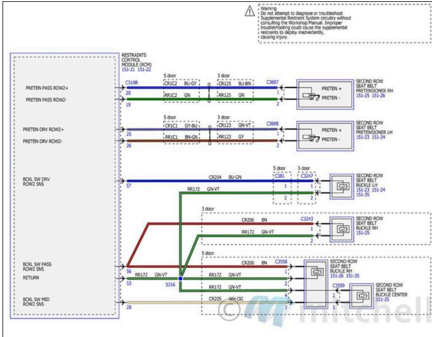
Fig. 195: Diagramas de cableado del sistema de retención suplementario (7 de 8)
