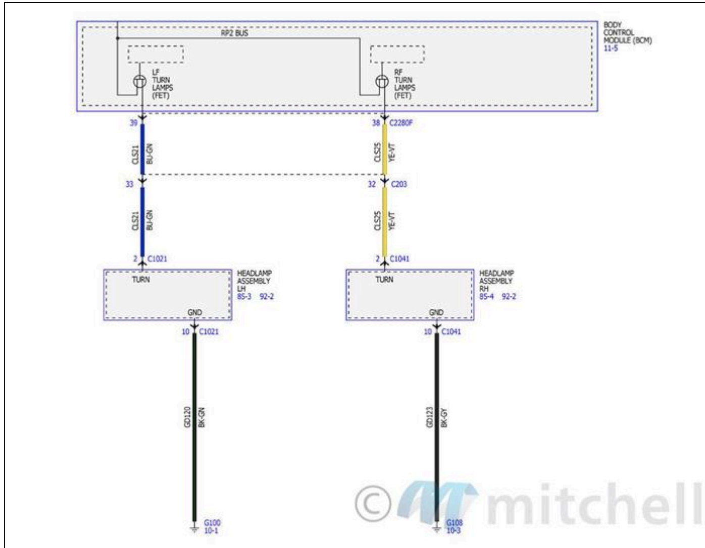
Fig. 209: Diagramas de cableado de luces de señal de giro, de freno y de emergencia (3 de 6)
