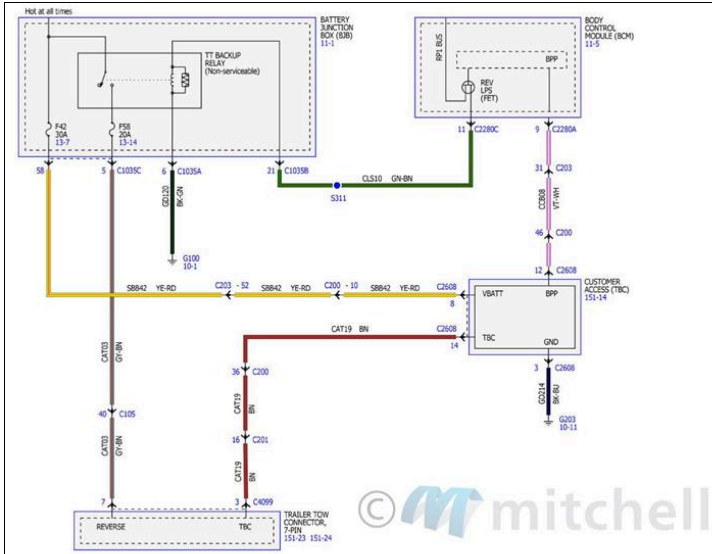
Fig. 199: Diagramas de cableado del adaptador de remolque/casa rodante (2 de 2)
