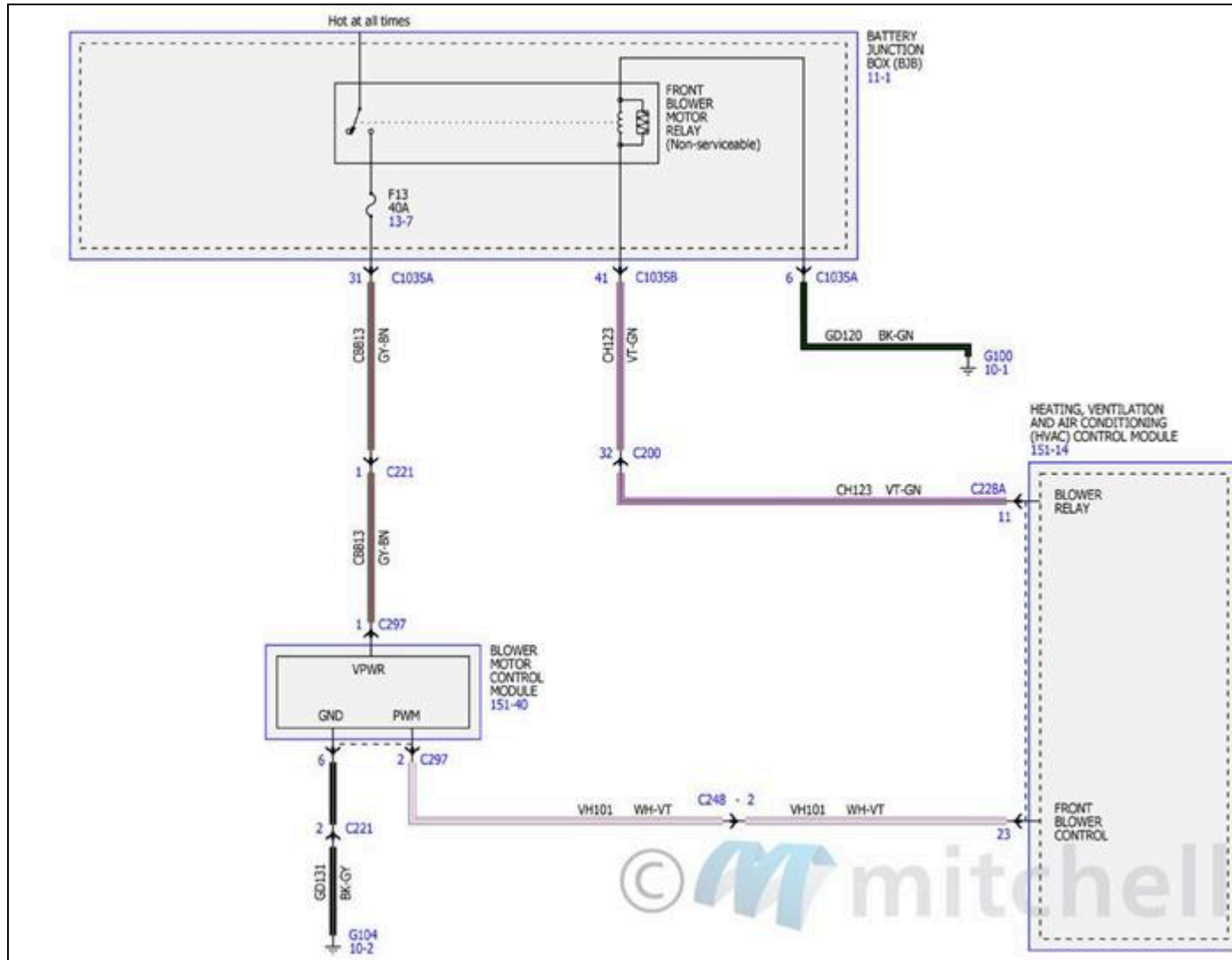
Fig. 16: Diagramas de cableado del sistema de control de clima automático (2 de 7)
