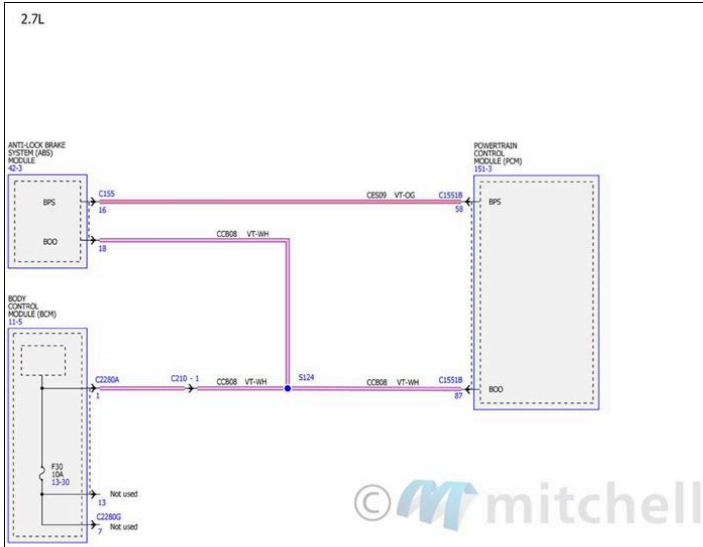
Fig. 38: Diagramas de cableado del control de crucero (7 de 7)
