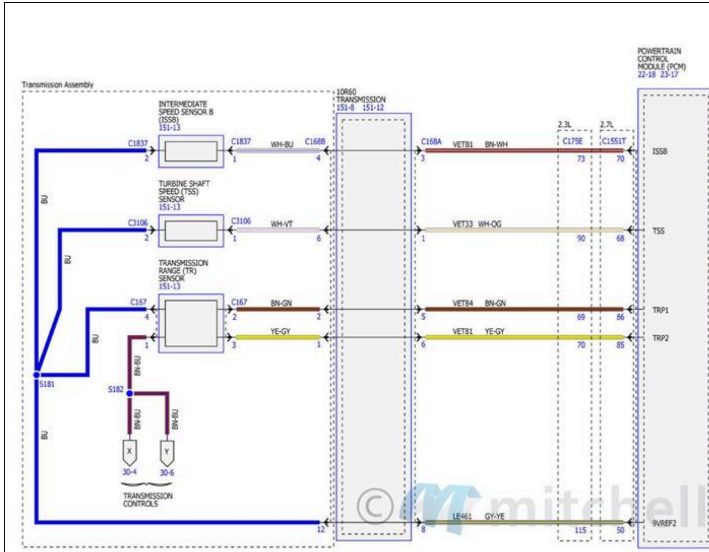
Fig. 202: Diagramas de cableado de los controles de transmisión - 10R60 (3 de 7)
