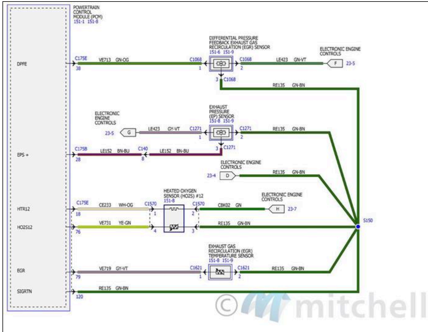
Fig. 48: Diagramas de cableado de los controles electrónicos del motor - 2.3L (6 de 17)
