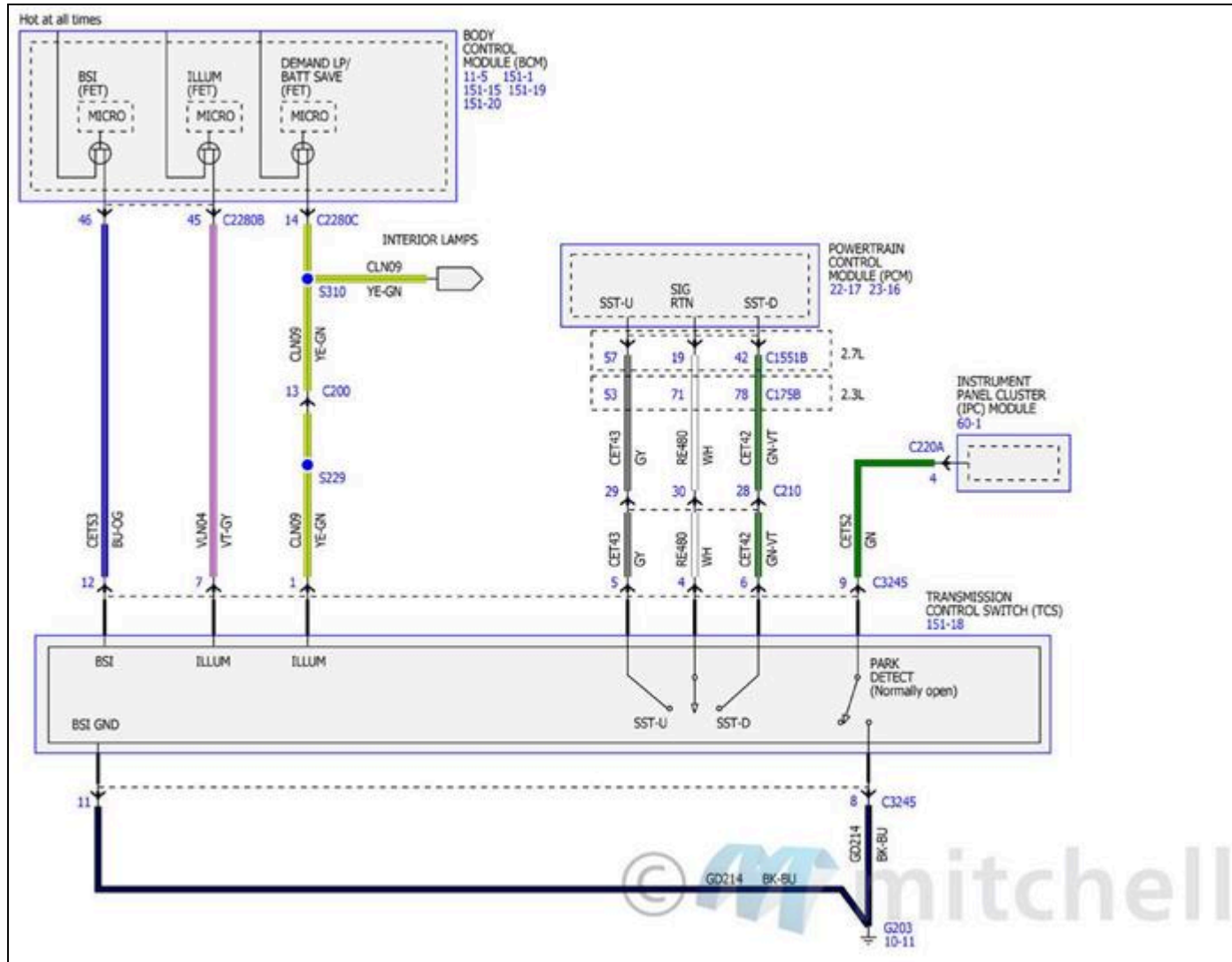
Fig. 206: Diagramas de cableado de los controles de transmisión - 10R60 (7 de 7)
