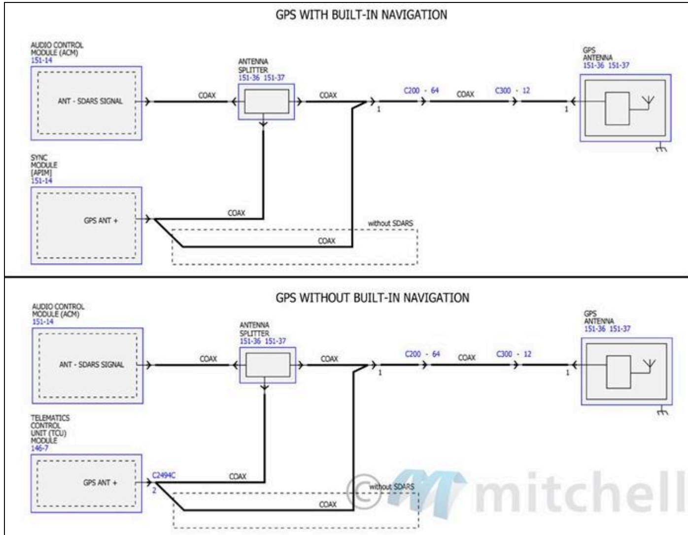
Fig. 14: Diagramas de cableado del sistema de audio (14 de 14)
