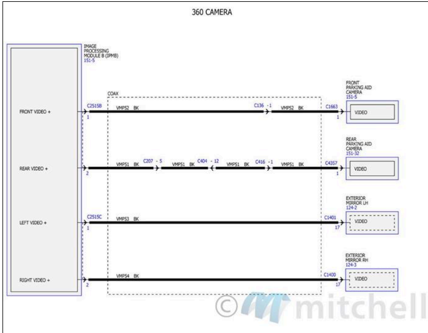
Fig. 223: Diagramas de cableado del sistema de mensajería de emergencia del vehículo (6 de 8)
