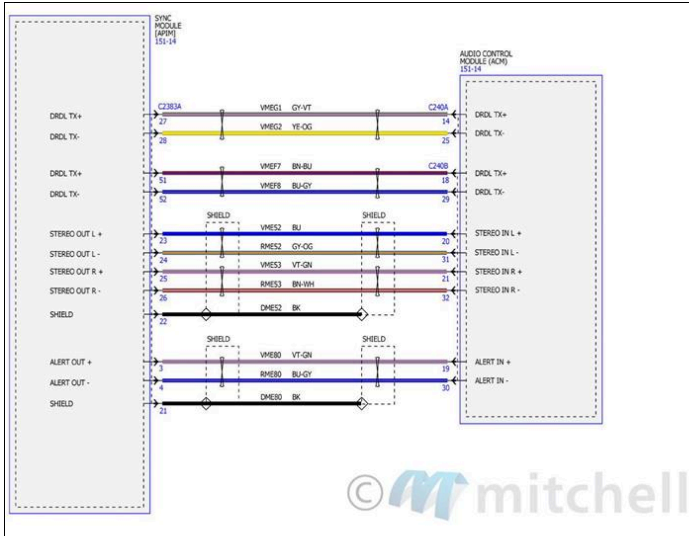
Fig. 5: Diagramas de cableado del sistema de audio (5 de 14)
