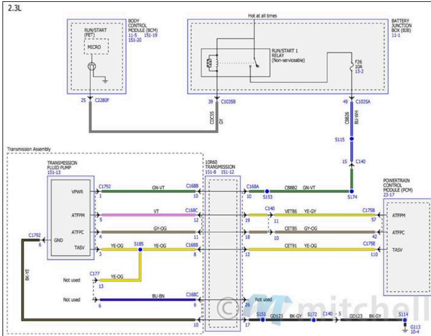
Fig. 201: Diagramas de cableado de los controles de transmisión - 10R60 (2 de 7)
