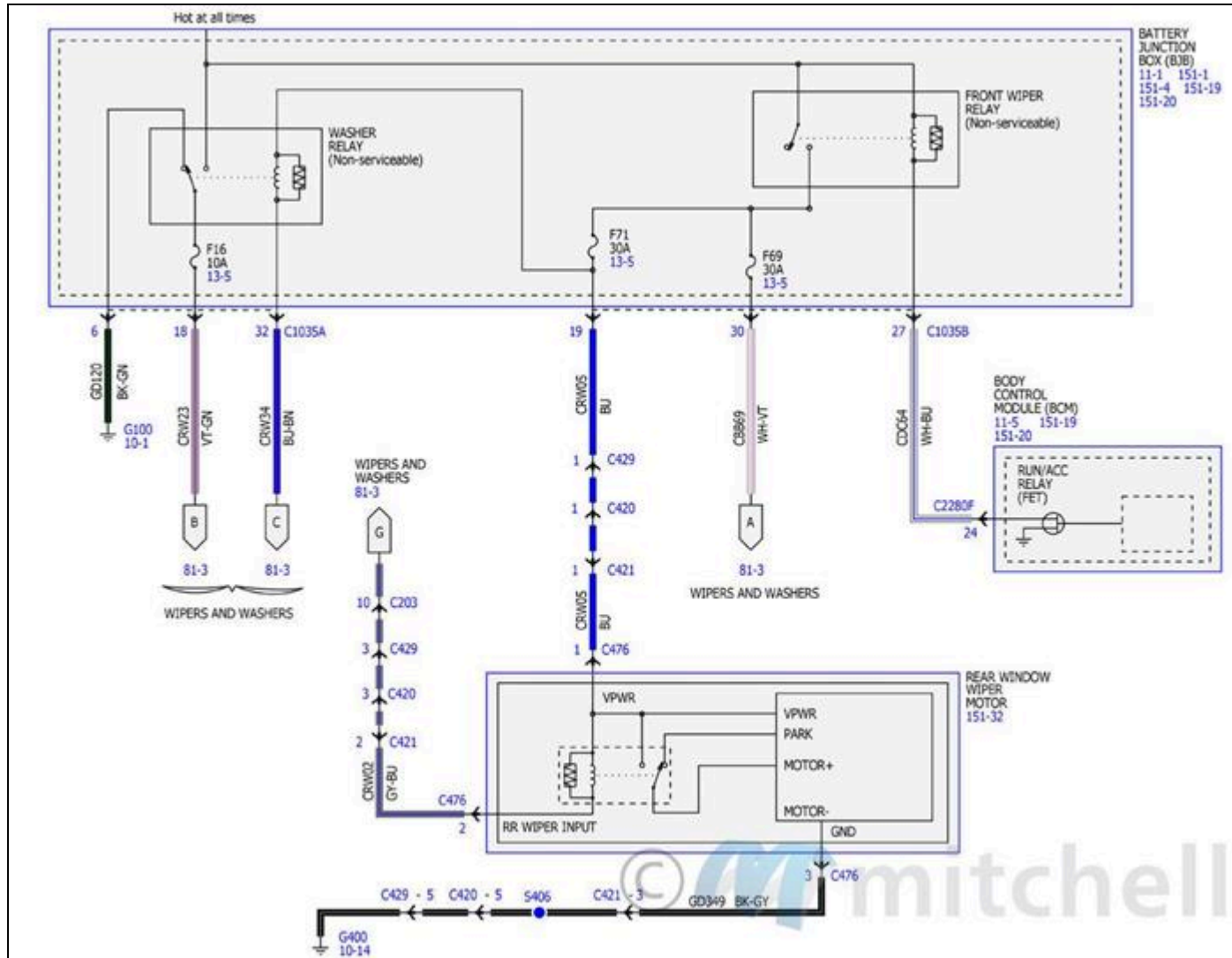
Fig. 227: Diagramas de cableado de limpiaparabrisas y lavaparabrisas (2 de 3)
