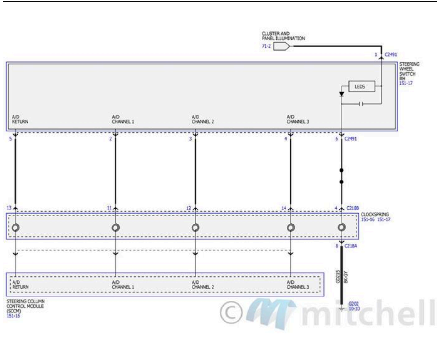
Fig. 12: Diagramas de cableado del sistema de audio (12 de 14)
