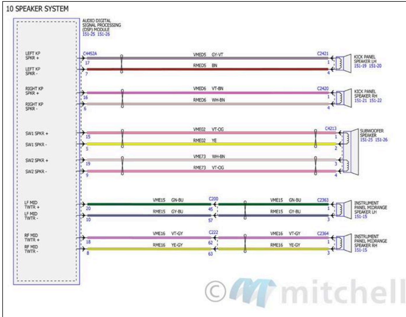
Fig. 9: Diagramas de cableado del sistema de audio (9 de 14)
