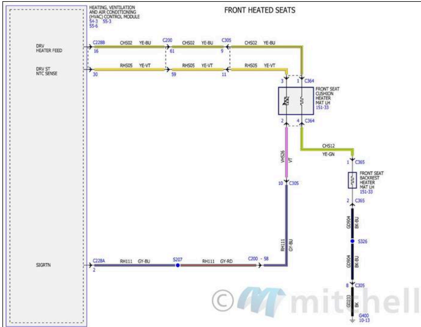
Fig. 24: Diagramas de cableado de asientos con control de clima (2 de 4)
