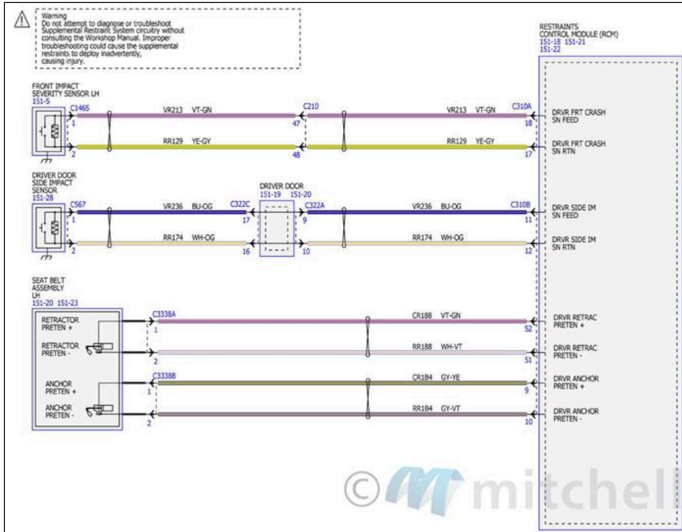
Fig. 191: Diagramas de cableado del sistema de retención suplementario (3 de 8)
