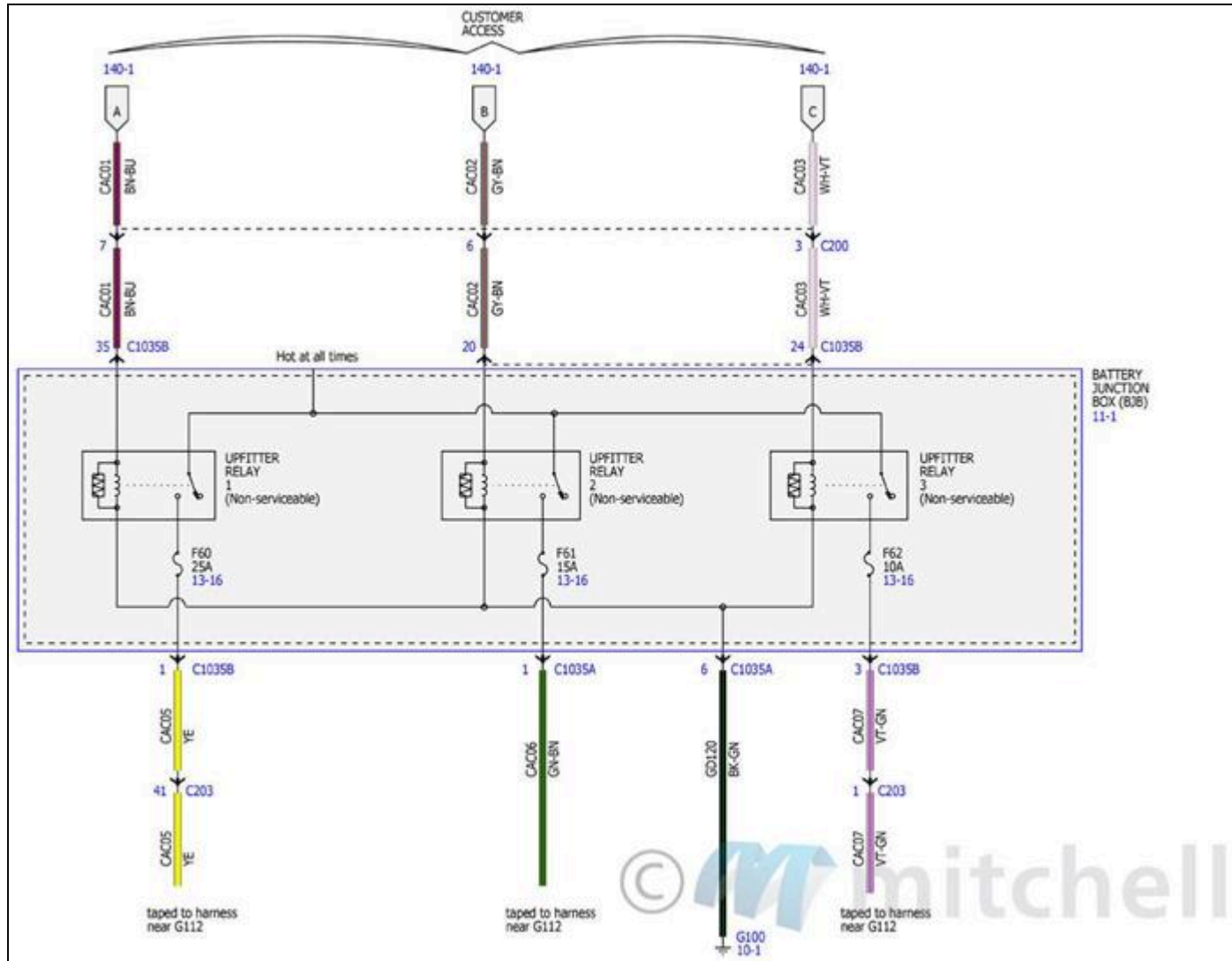
Fig. 40: Diagramas de cableado de acceso del cliente (2 de 4)
