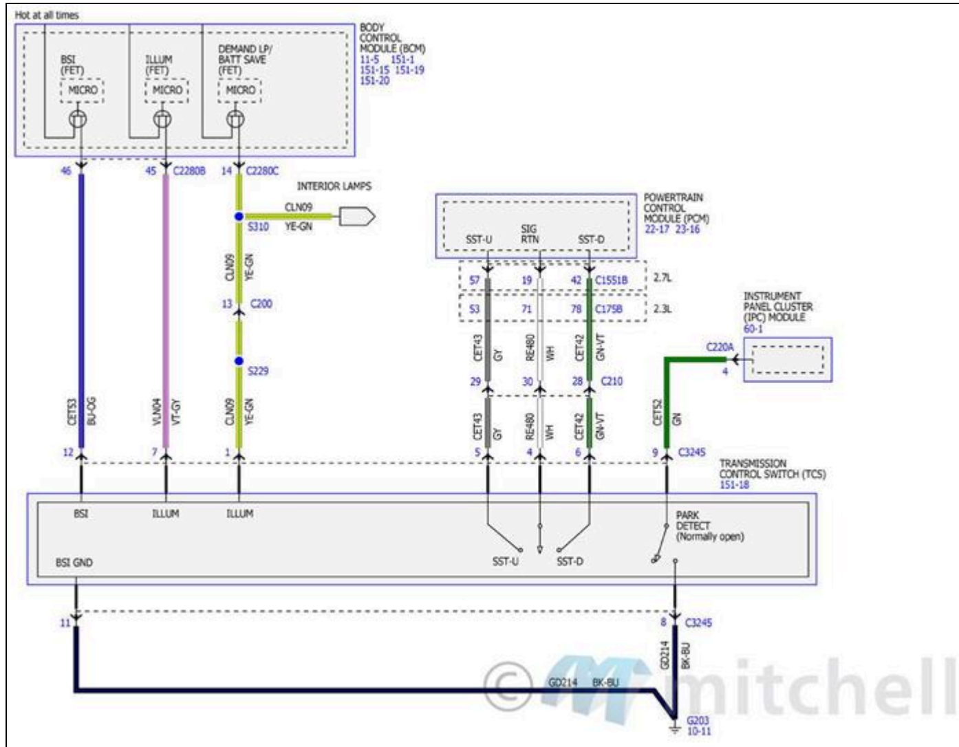
Fig. 186: Shift Interlock Wiring Diagram
