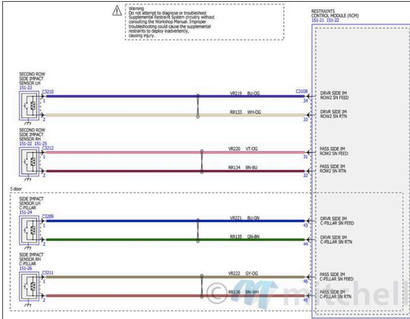
Fig. 193: Diagramas de cableado del sistema de retención suplementario (5 de 8)
