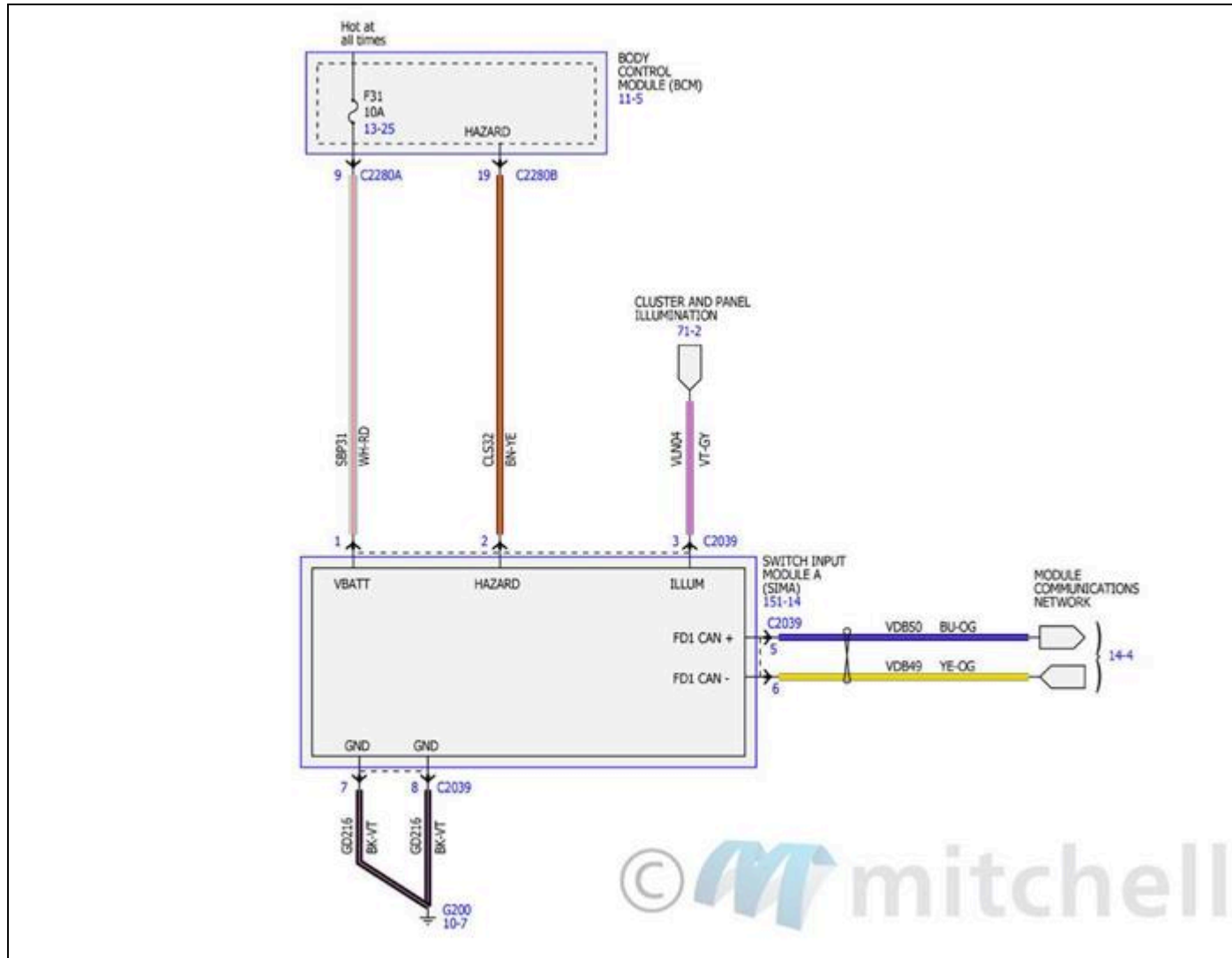
Fig. 208: Diagramas de cableado de luces de señal de giro, de freno y de emergencia (2 de 6)
