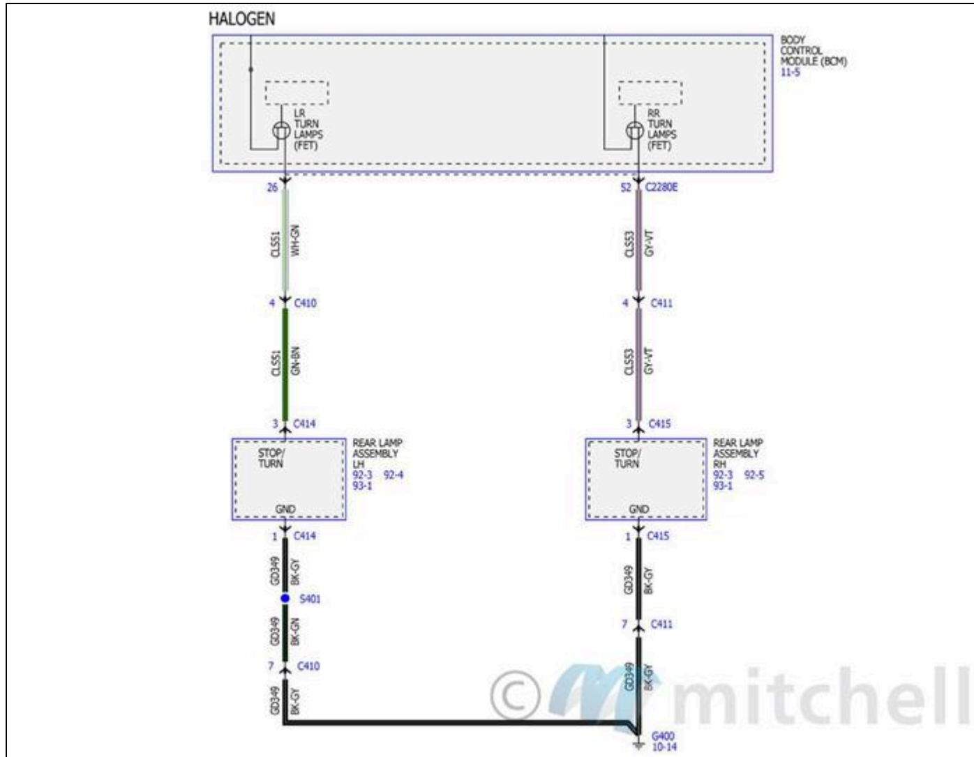
Fig. 210: Diagramas de cableado de luces de giro, de freno y de emergencia (4 de 6)
