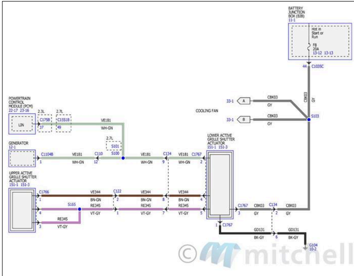
Fig. 31: Diagramas de cableado del ventilador de enfriamiento (2 de 2)
