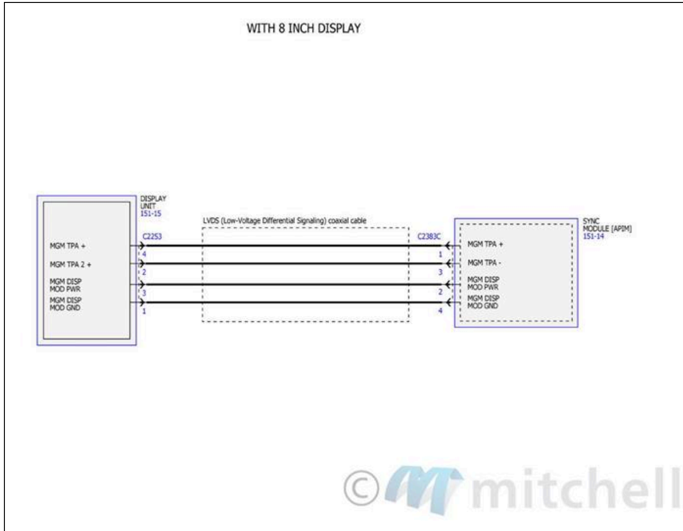
Fig. 4: Diagramas de cableado del sistema de audio (4 de 14)
