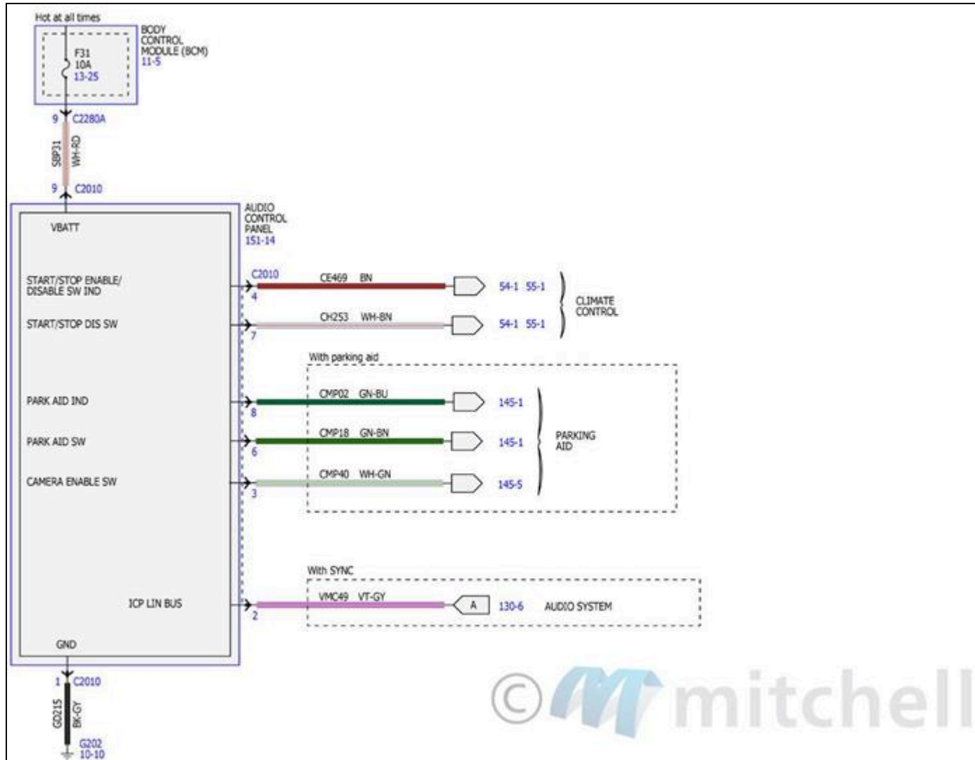
Fig. 13: Diagramas de cableado del sistema de audio (13 de 14)
