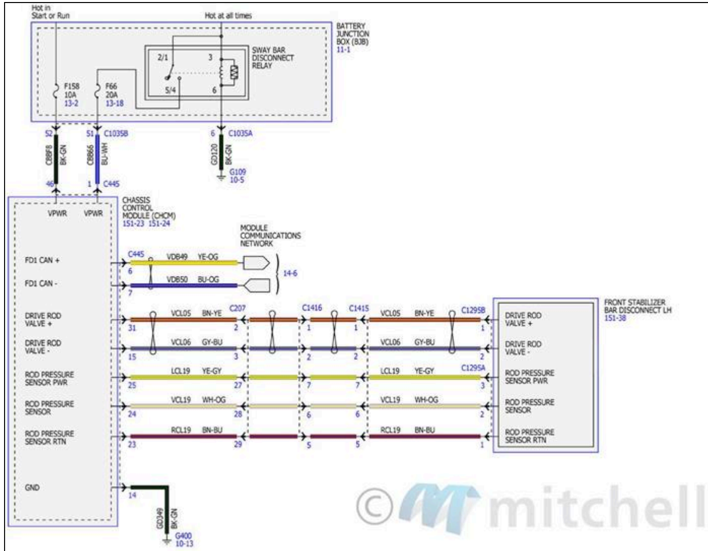
Fig. 213: Diagramas de cableado de la suspensión dinámica del vehículo (1 de 2)
