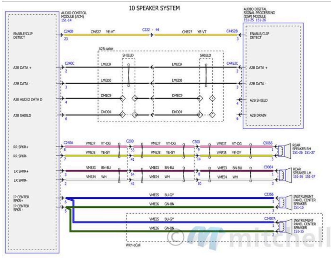
Fig. 7: Diagramas de cableado del sistema de audio (7 de 14)
