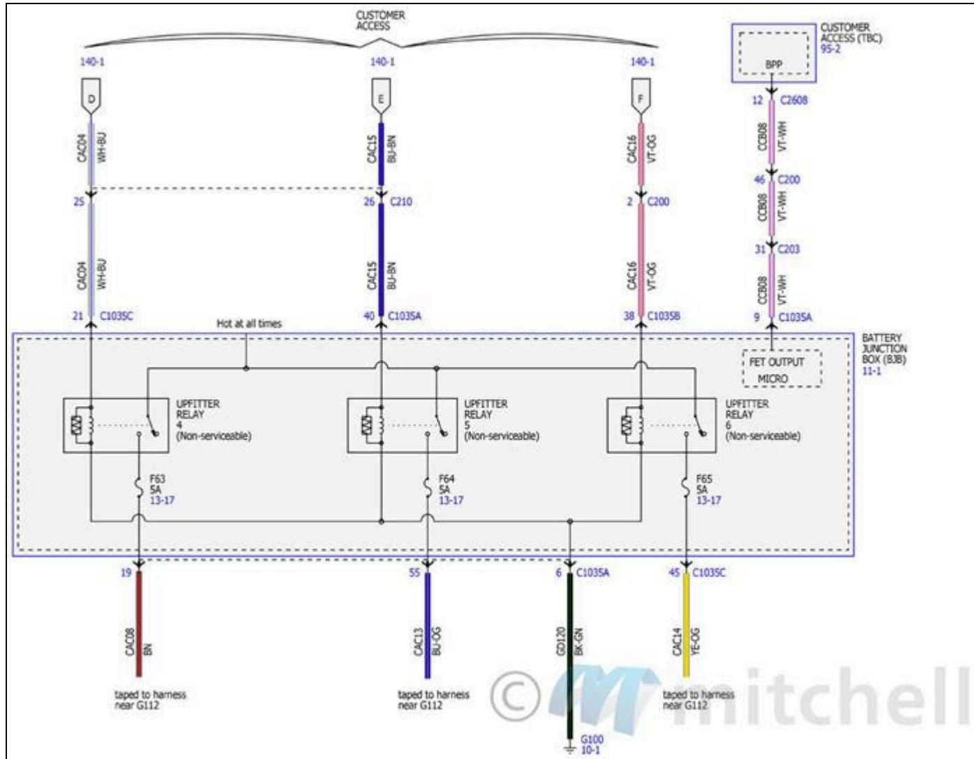
Fig. 41: Diagramas de cableado de acceso del cliente (3 de 4)
