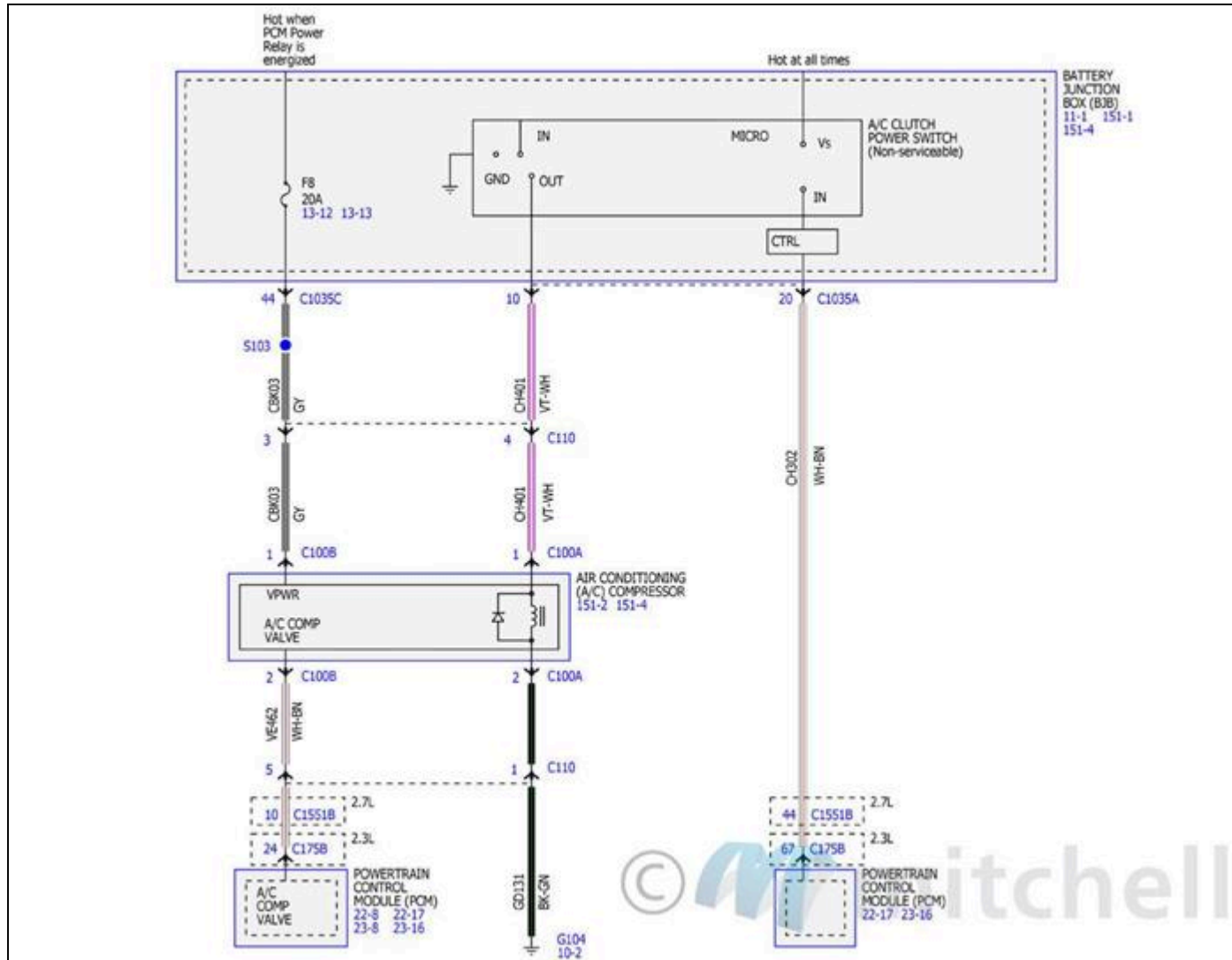
Fig. 21: Diagramas de cableado del sistema de control de clima automático (7 de 7)
