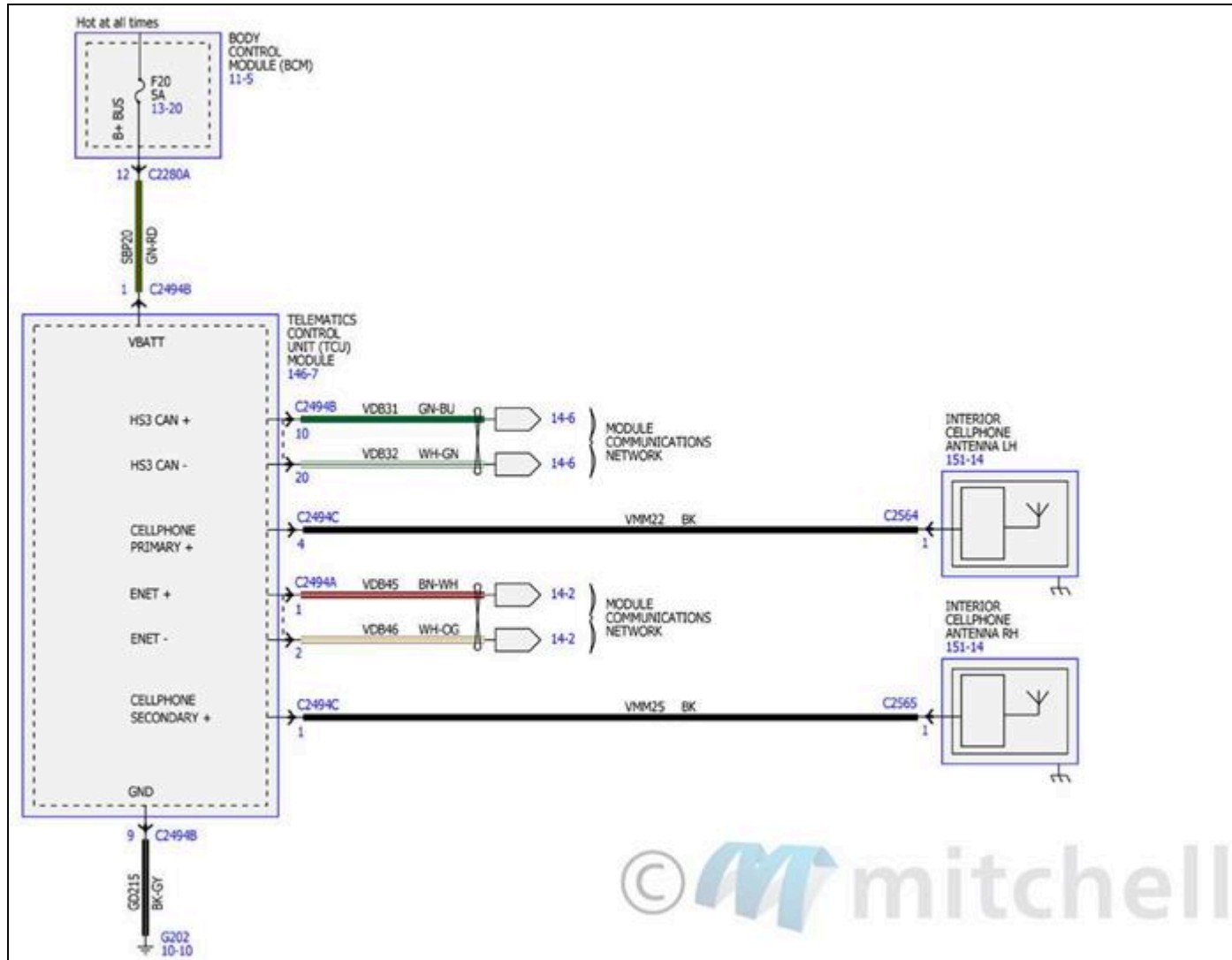
Fig. 224: Diagramas de cableado del sistema de mensajería de emergencia del vehículo (7 de 8)
