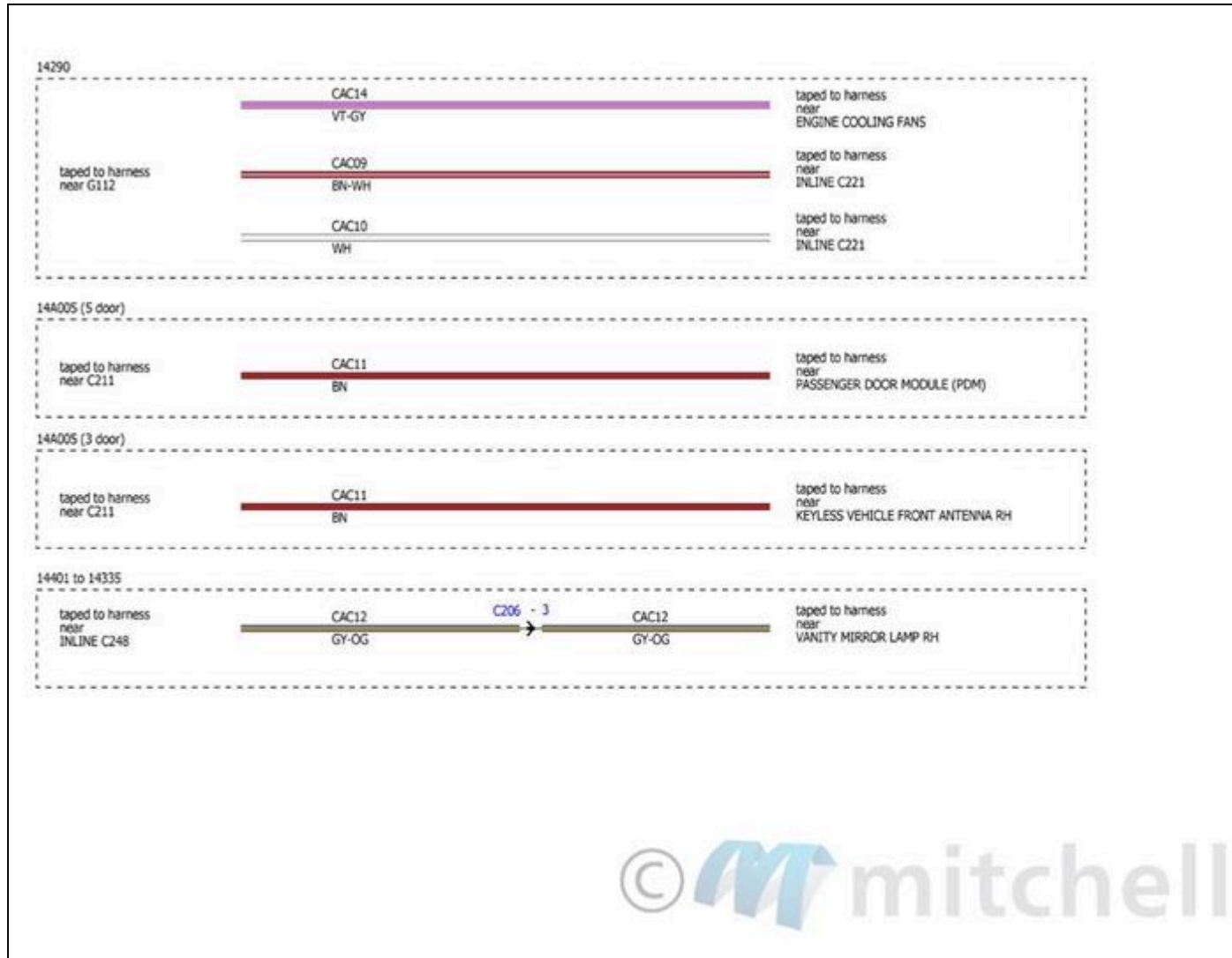
Fig. 42: Diagramas de cableado de acceso del cliente (4 de 4)
