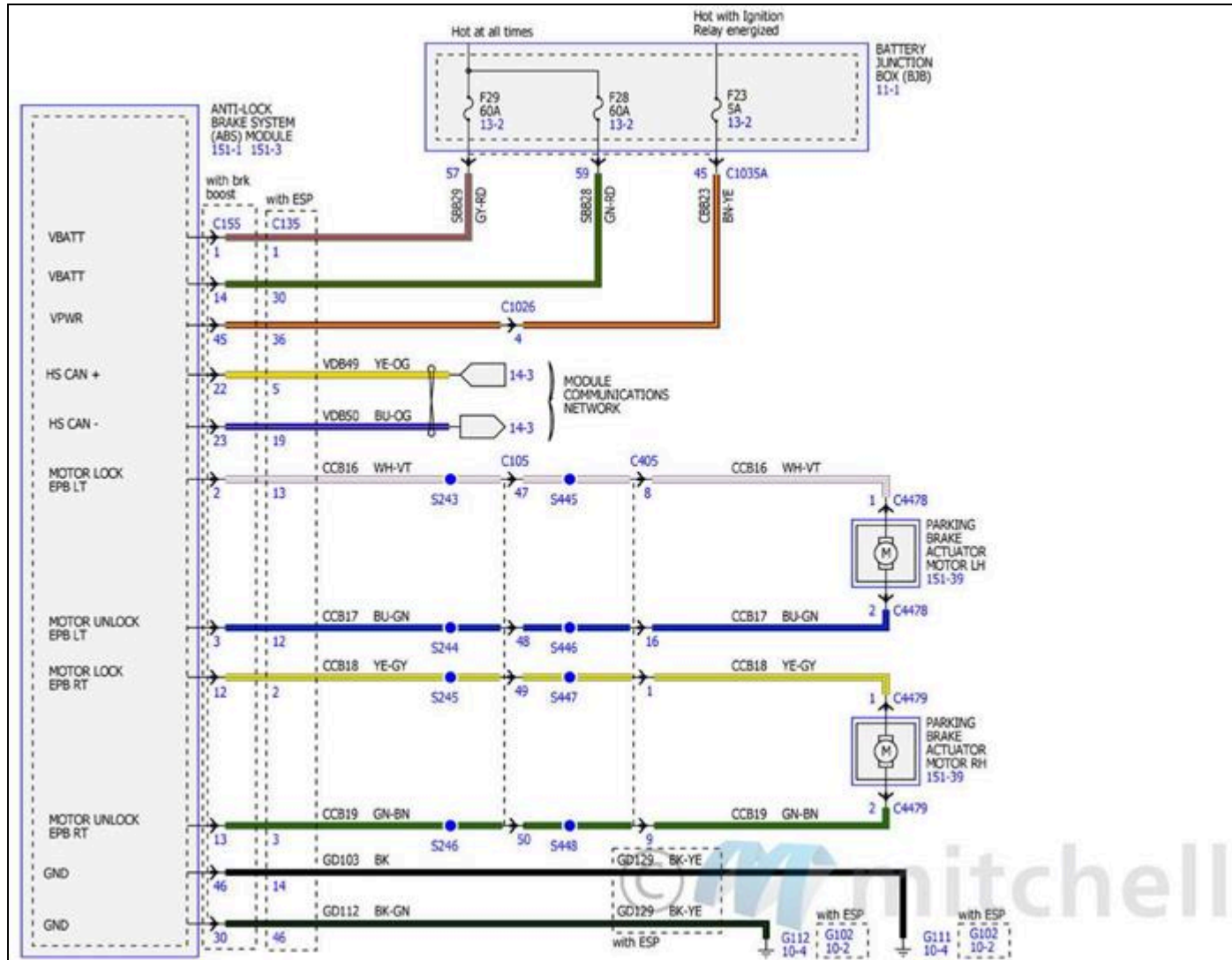
Fig. 215: Diagramas de cableado de los sistemas dinámicos del vehículo (1 de 3)
