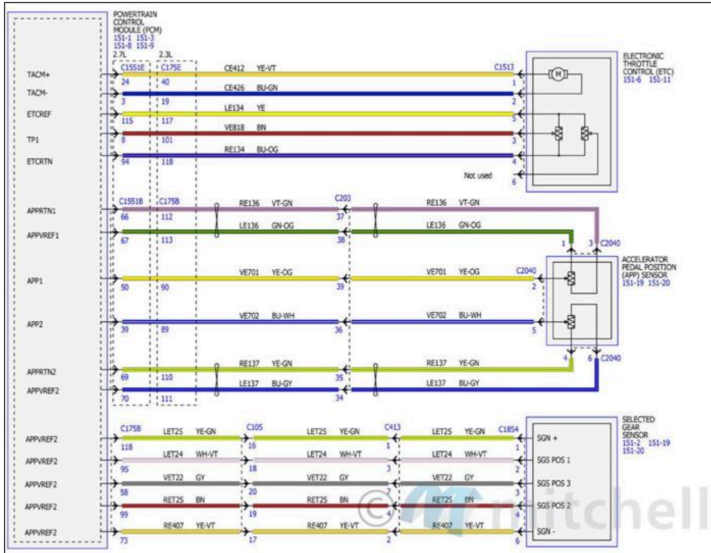
Fig. 35: Diagramas de cableado del control de crucero (4 de 7)
