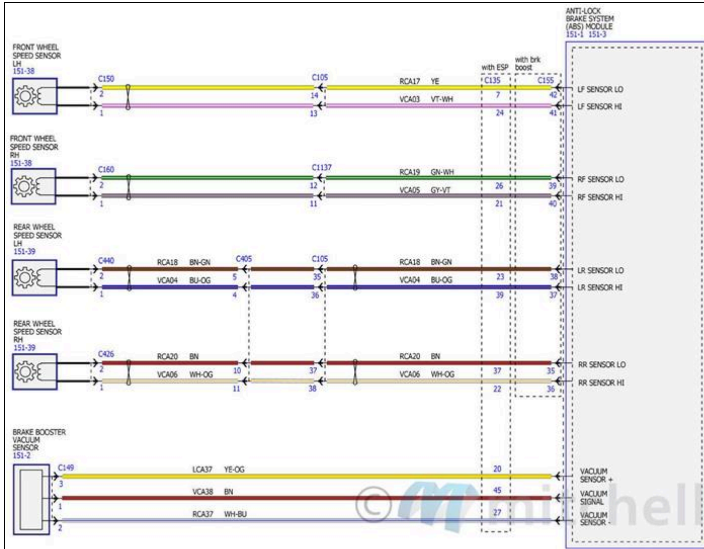
Fig. 216: Diagramas de cableado de los sistemas dinámicos del vehículo (2 de 3)
