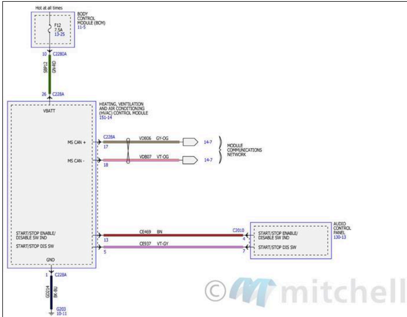
Fig. 15: Diagramas de cableado del sistema de control de clima automático (1 de 7)
