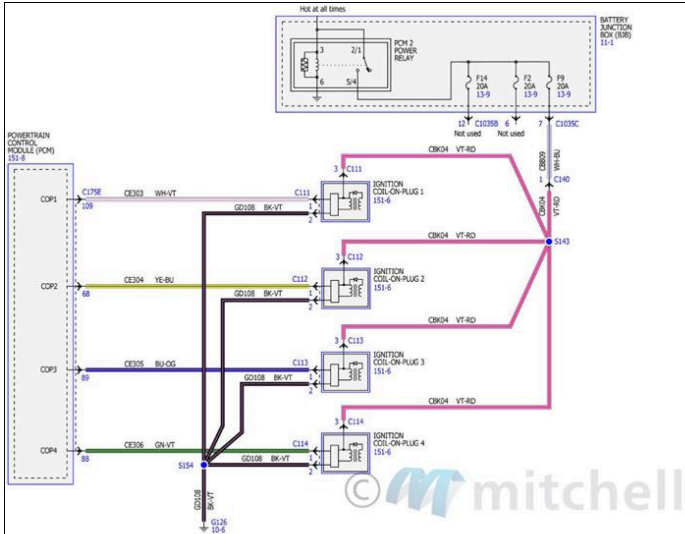
Fig. 44: Diagramas de cableado de los controles electrónicos del motor - 2.3L (2 de 17)
