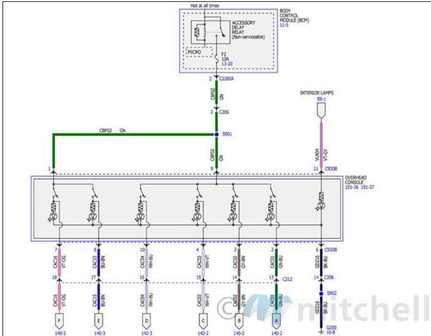
Fig. 39: Diagramas de cableado de acceso del cliente (1 de 4)
