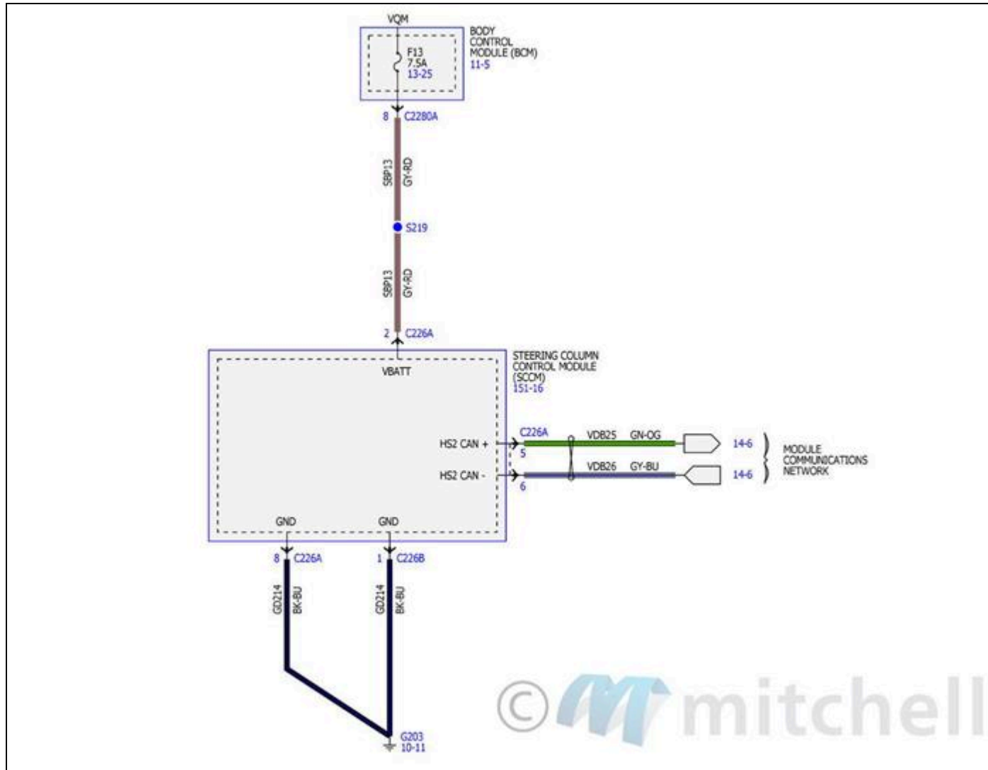
Fig. 32: Diagramas de cableado del control de crucero (1 de 7)
