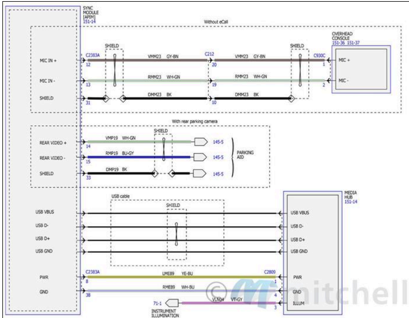
Fig. 10: Diagramas de cableado del sistema de audio (10 de 14)
