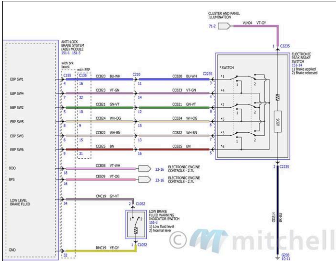
Fig. 217: Diagramas de cableado de sistemas dinámicos del vehículo (3 de 3)
