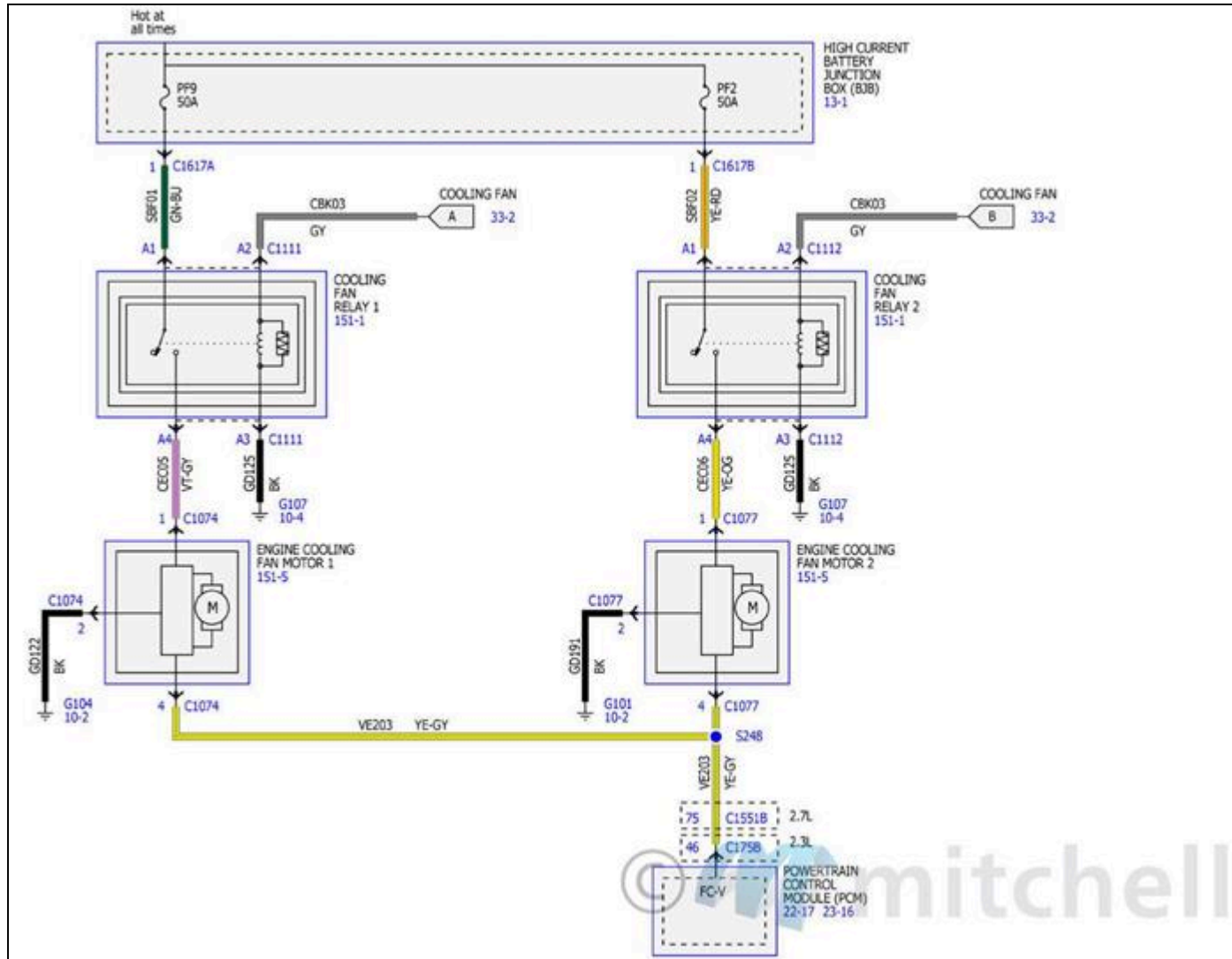
Fig. 30: Diagramas de cableado del ventilador de enfriamiento (1 de 2)
