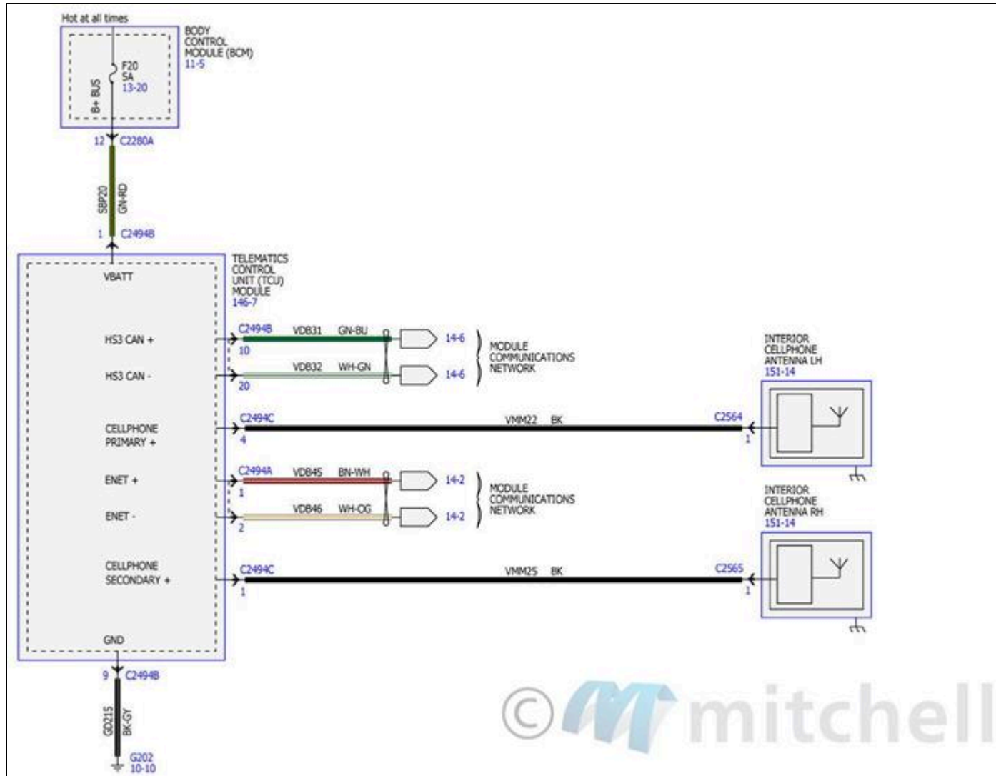
Fig. 11: Diagramas de cableado del sistema de audio (11 de 14)
