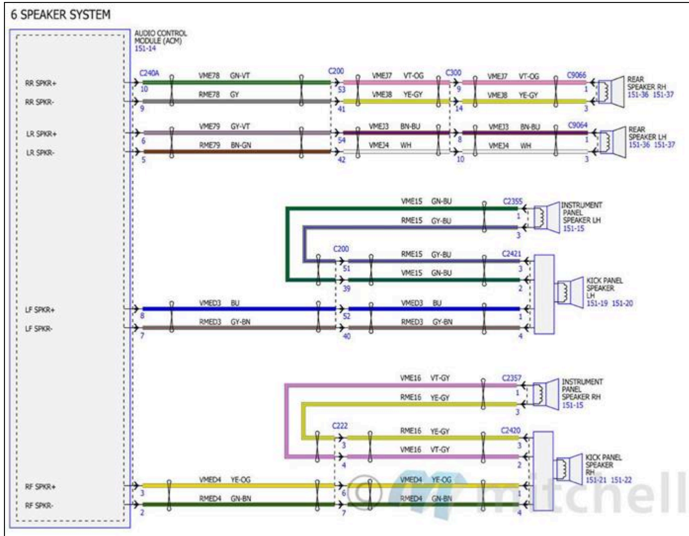
Fig. 2: Diagramas de cableado del sistema de audio (2 de 14)
