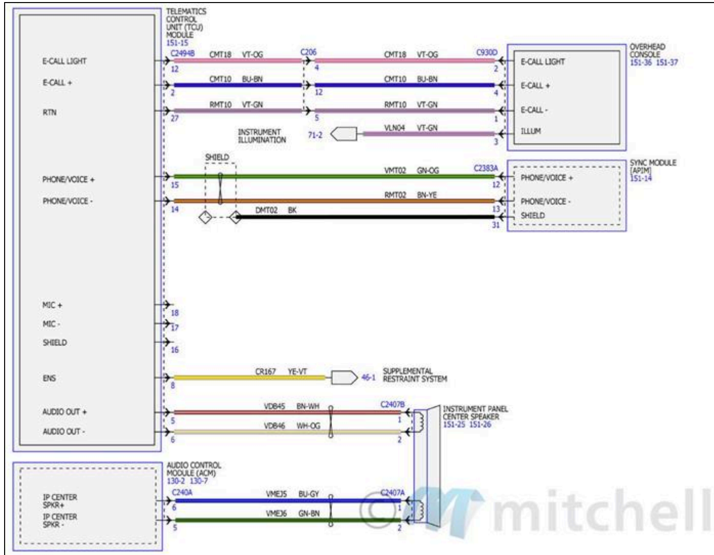
Fig. 225: Diagramas de cableado del sistema de mensajería de emergencia del vehículo (8 de 8)
