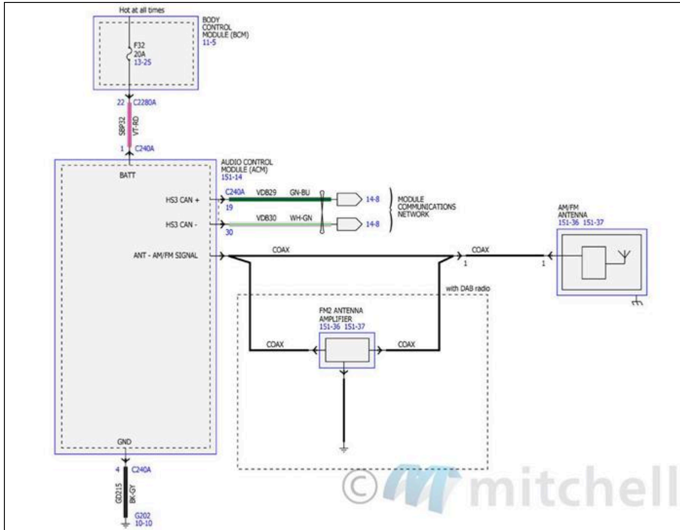
Fig. 1: Diagramas de cableado del sistema de audio (1 de 14)
