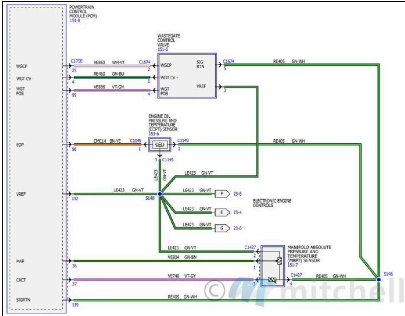
Fig. 47: Diagramas de cableado de los controles electrónicos del motor - 2.3L (5 de 17)
