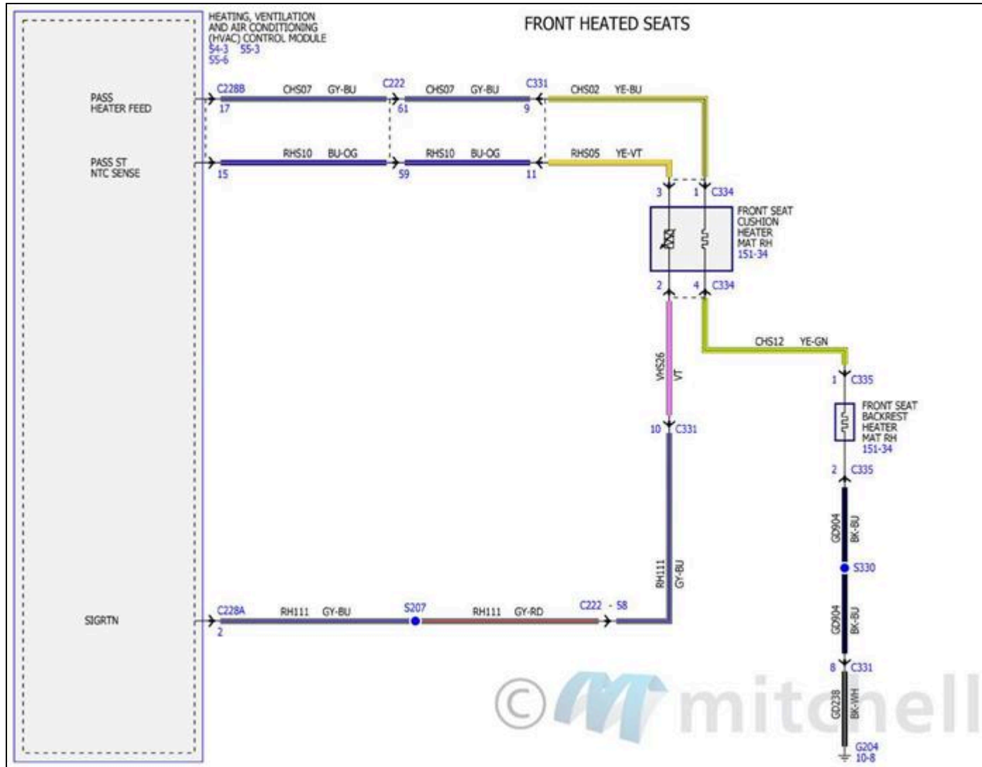
Fig. 25: Diagramas de cableado de asientos con control de clima (3 de 4)
