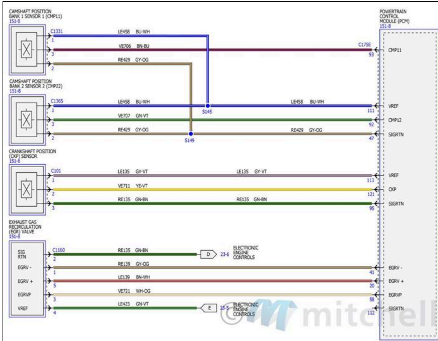
Fig. 46: Diagramas de cableado de los controles electrónicos del motor - 2.3L (4 de 17)
