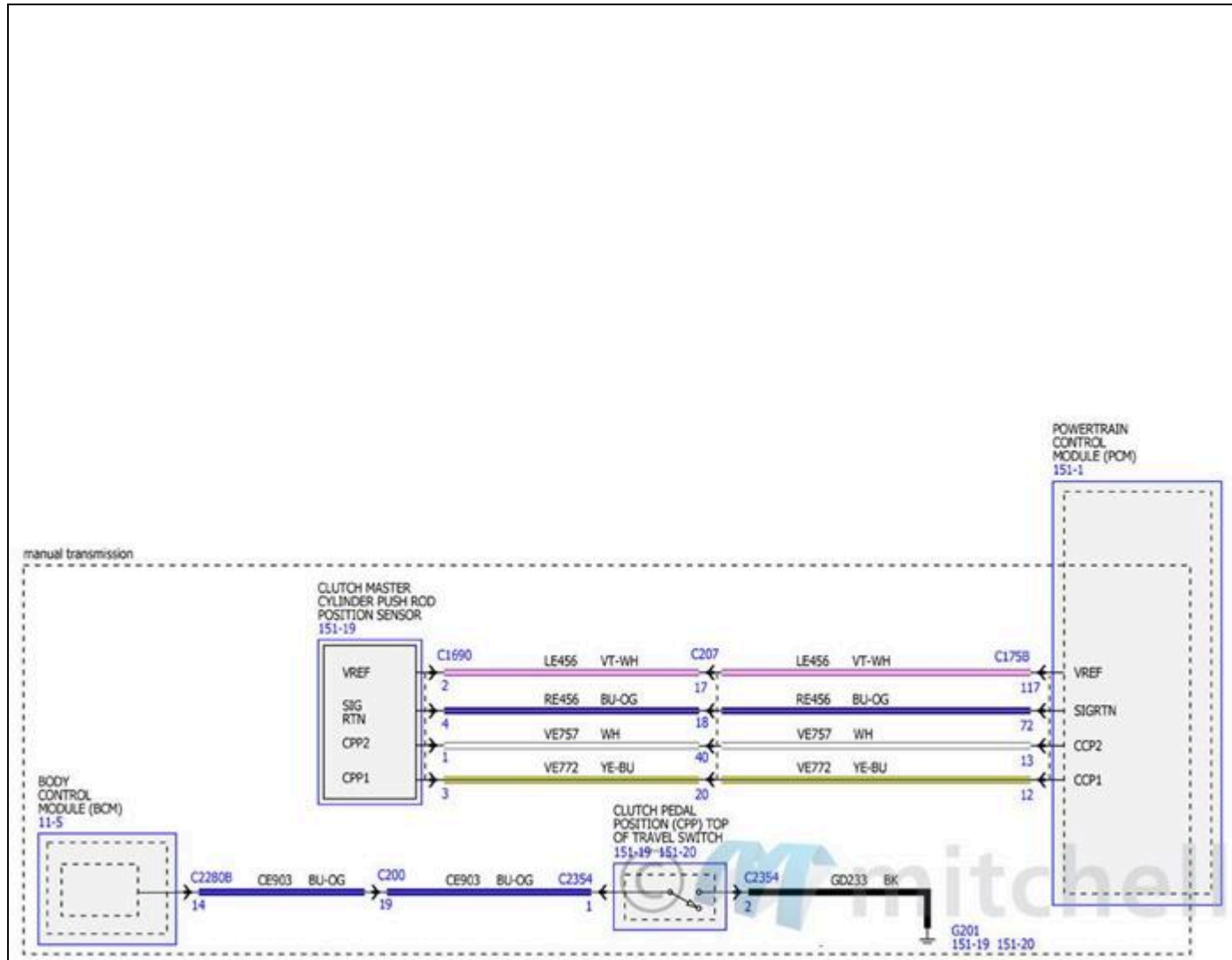
Fig. 37: Diagramas de cableado del control de crucero (6 de 7)
