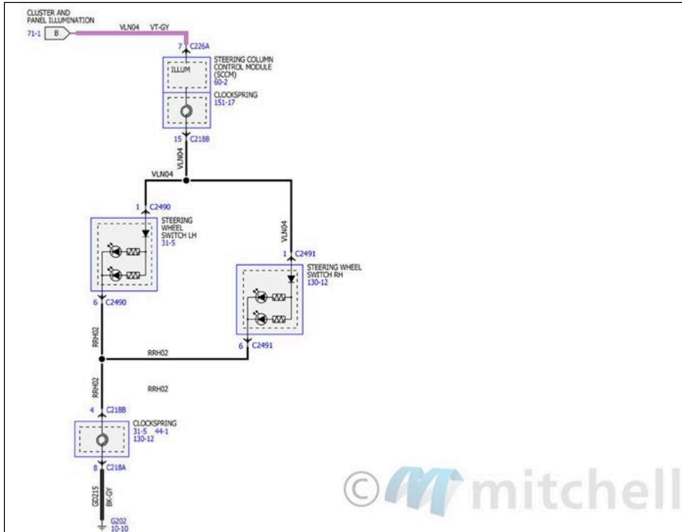
Fig. 29: Diagramas de cableado de iluminación de grupos y paneles (3 de 3)
