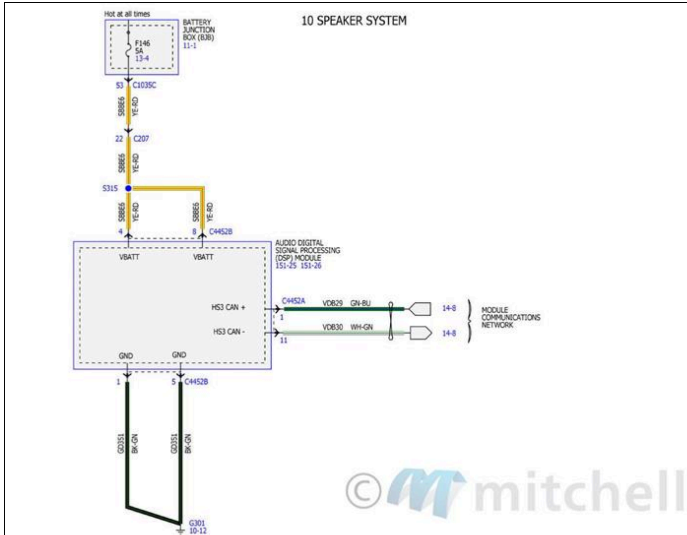
Fig. 8: Diagramas de cableado del sistema de audio (8 de 14)
