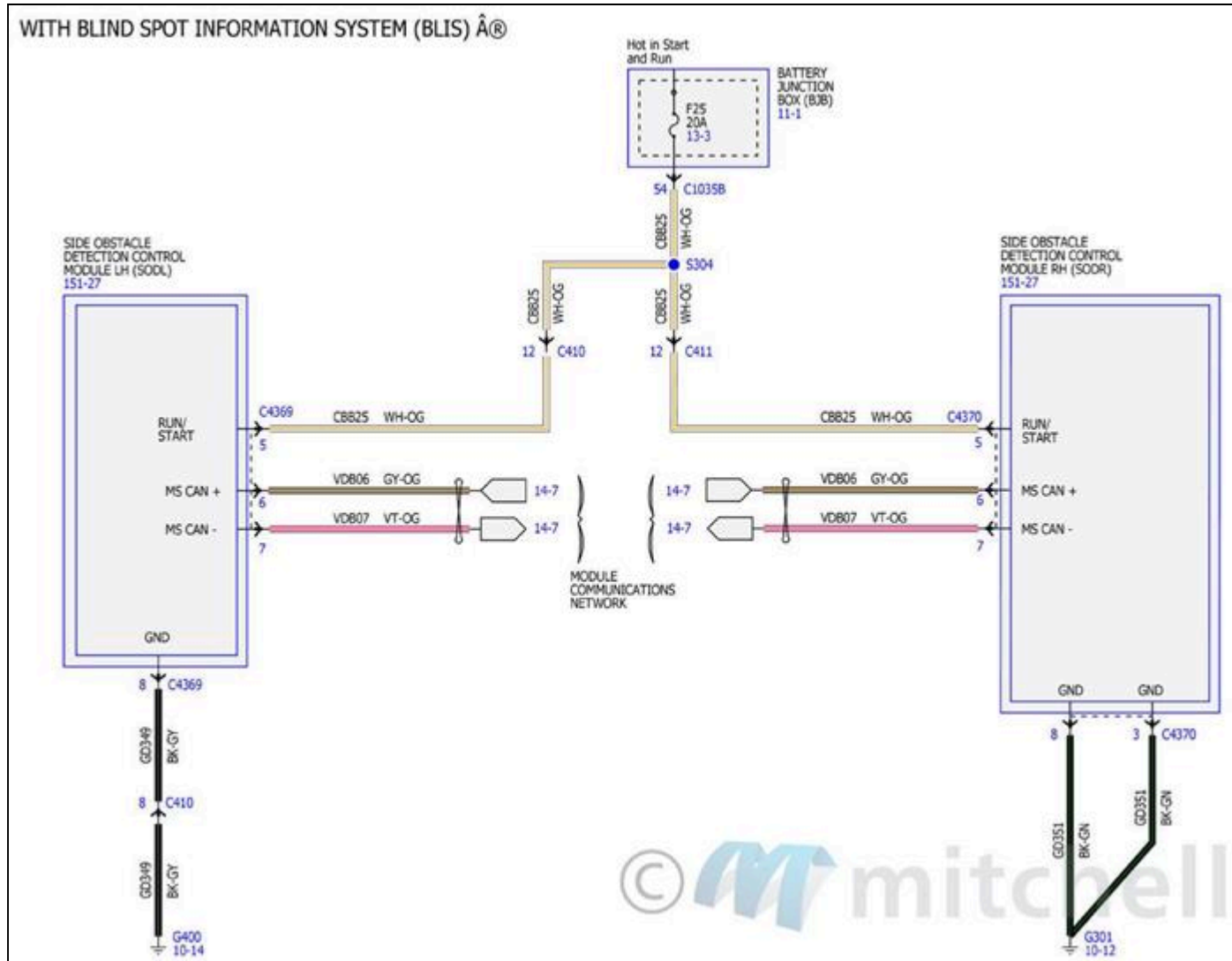
Fig. 219: Diagramas de cableado del sistema de mensajería de emergencia del vehículo (2 de 8)
