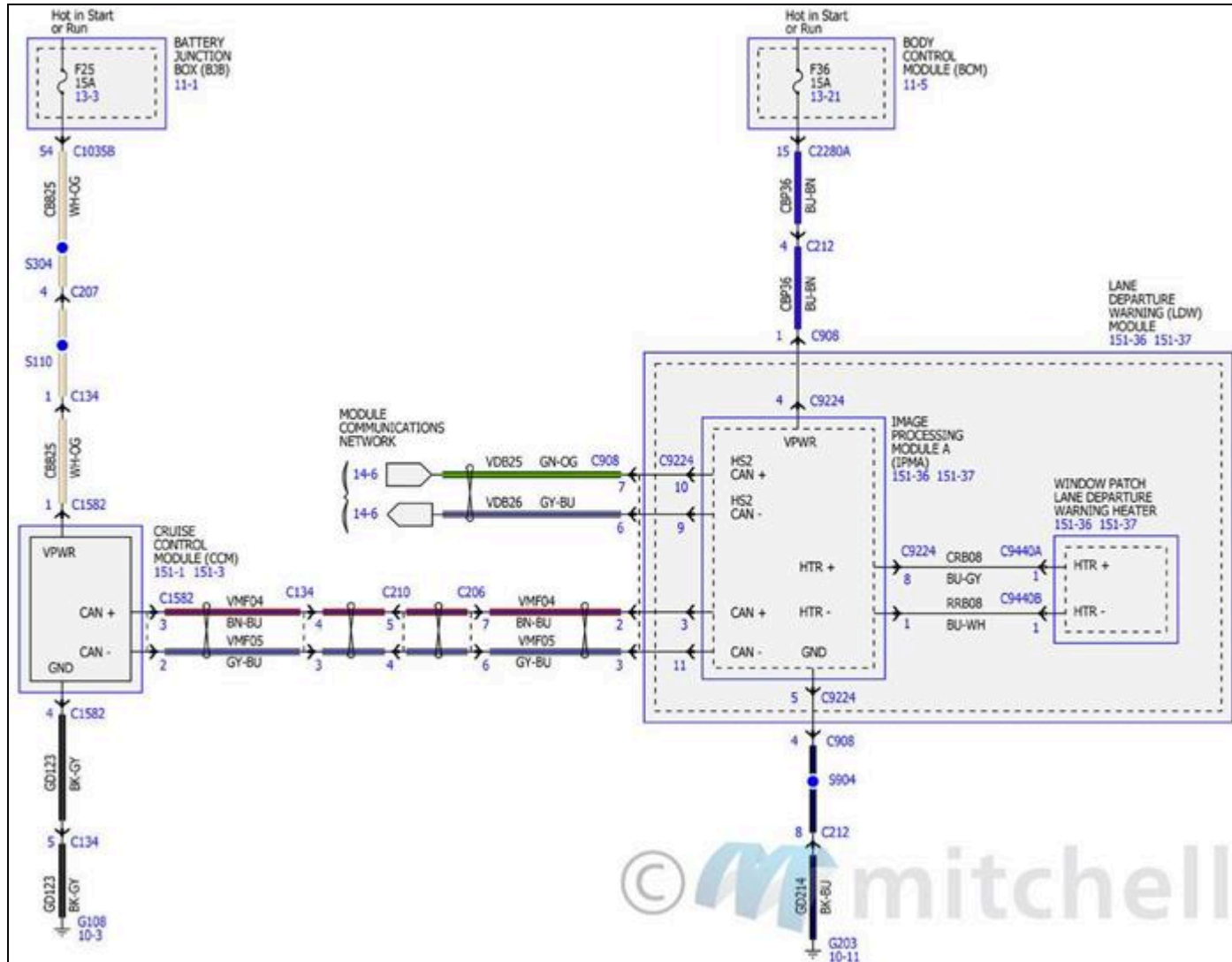
Fig. 33: Diagramas de cableado del control de crucero (2 de 7)
