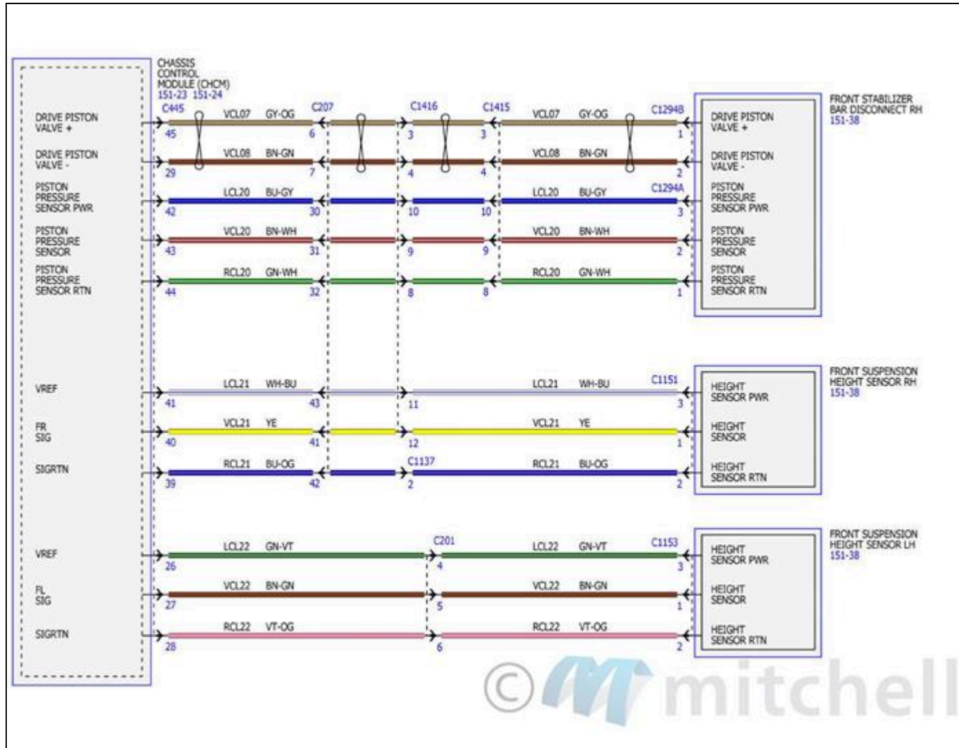
Fig. 214: Diagramas de cableado de la suspensión dinámica del vehículo (2 de 2)
