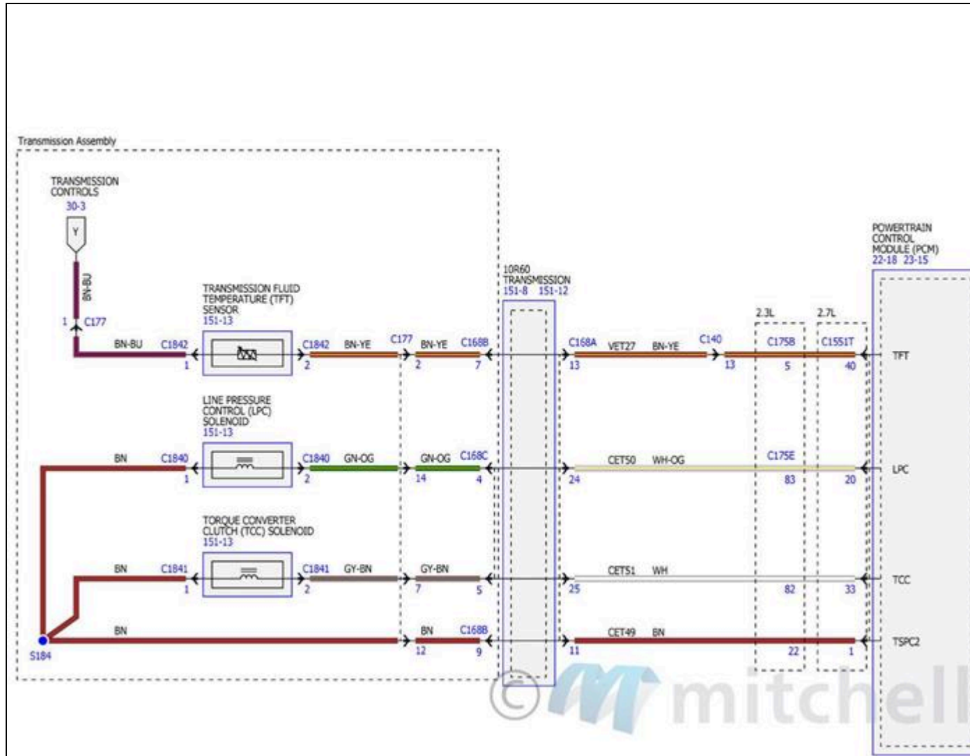
Fig. 205: Diagramas de cableado de los controles de transmisión - 10R60 (6 de 7)
