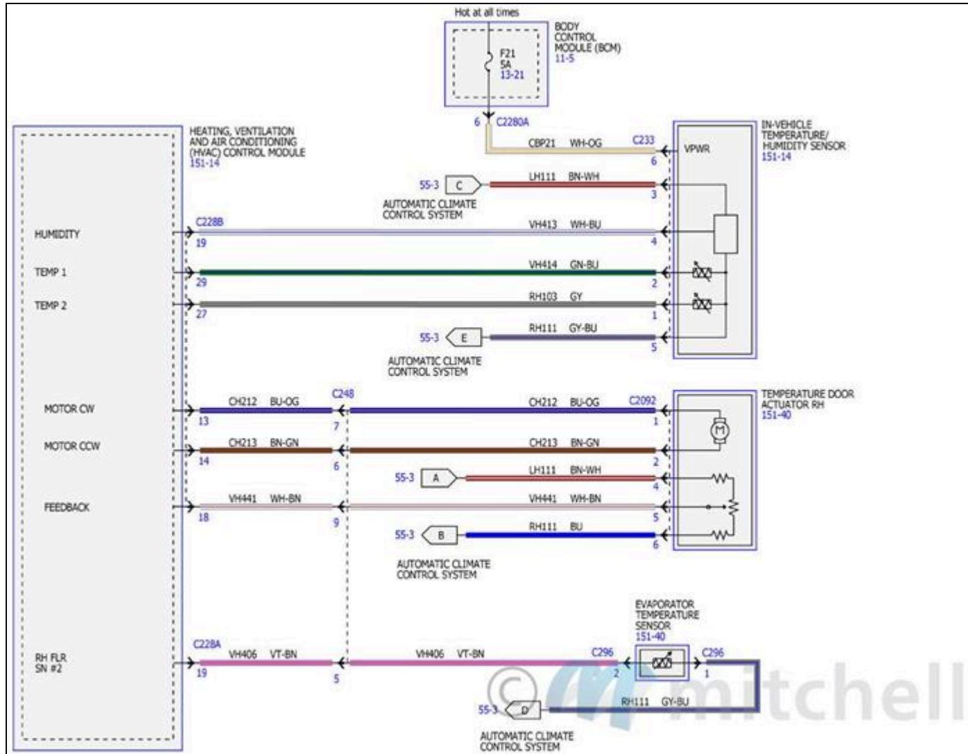
Fig. 18: Diagramas de cableado del sistema de control de clima automático (4 de 7)
