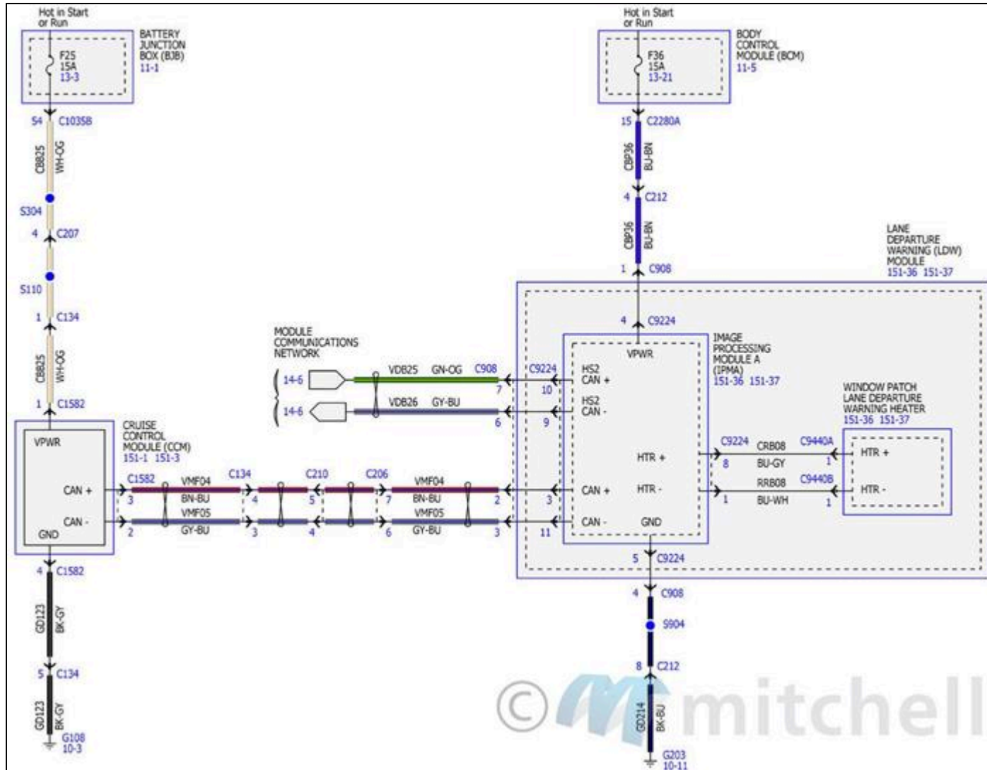
Fig. 218: Diagramas de cableado del sistema de mensajería de emergencia del vehículo (1 de 8)
