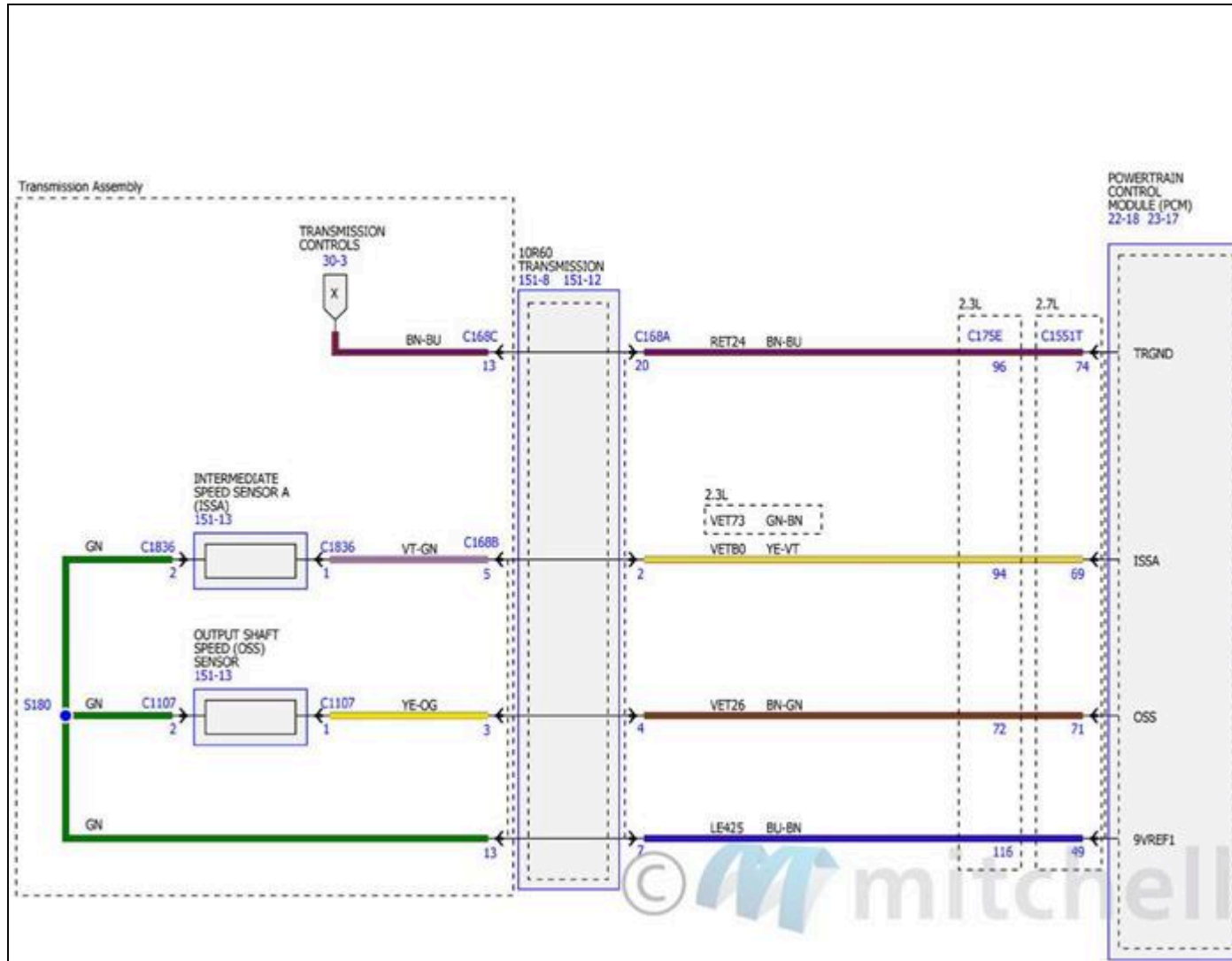
Fig. 203: Diagramas de cableado de los controles de transmisión - 10R60 (4 de 7)
