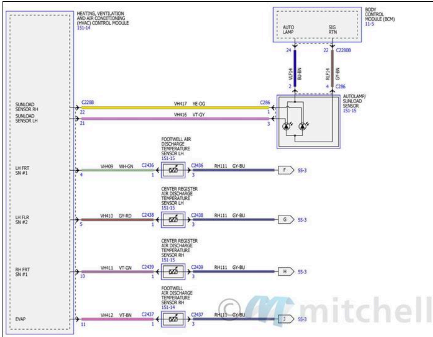
Fig. 19: Diagramas de cableado del sistema de control de clima automático (5 de 7)
