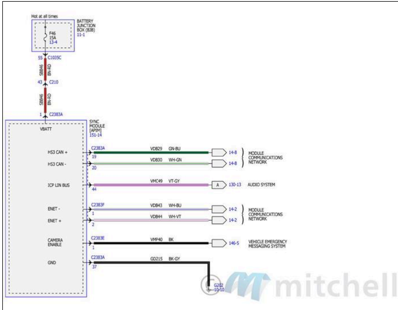
Fig. 6: Diagramas de cableado del sistema de audio (6 de 14)
