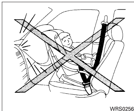
INSTALLATION D'UN DISPOSITIF DE RETENUE POUR ENFANT ORIENTÉ VERS L'ARRIÈRE À L'AIDE DES CEINTURES DE SÉCURITÉ
