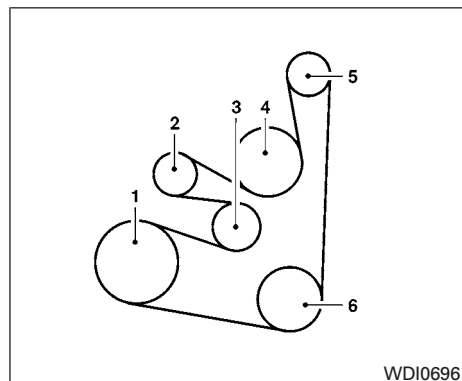
Modèle QR25DE
