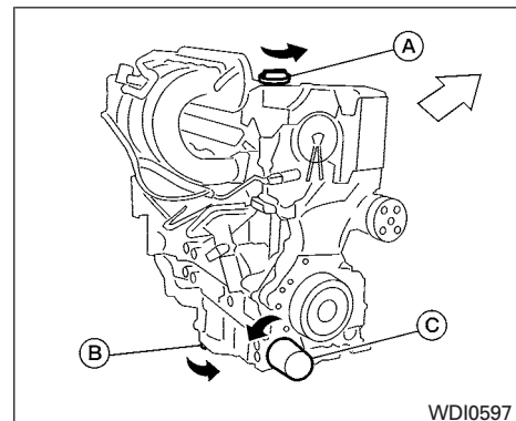
Moteur QR25DE
