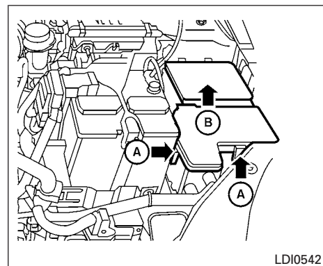
Moteur MR20DE
