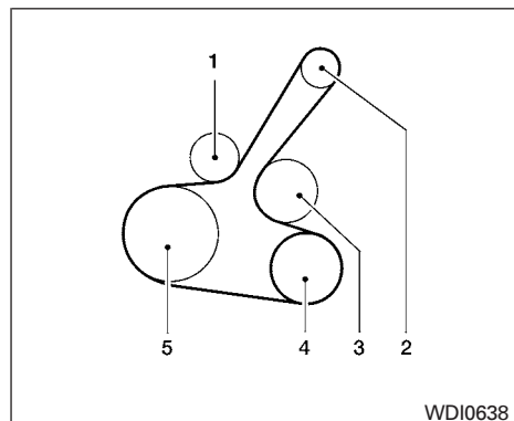
Modèle MR20DE
