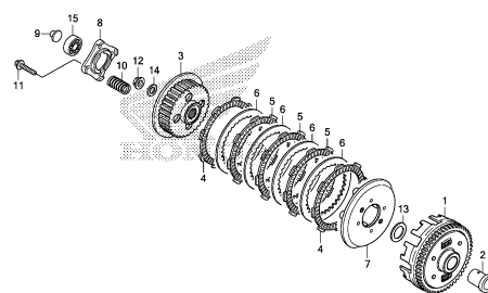
CLUTCH
