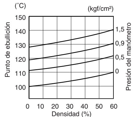
Fig. 2 Curva de densidad del refrigerante-punto de ebullición
