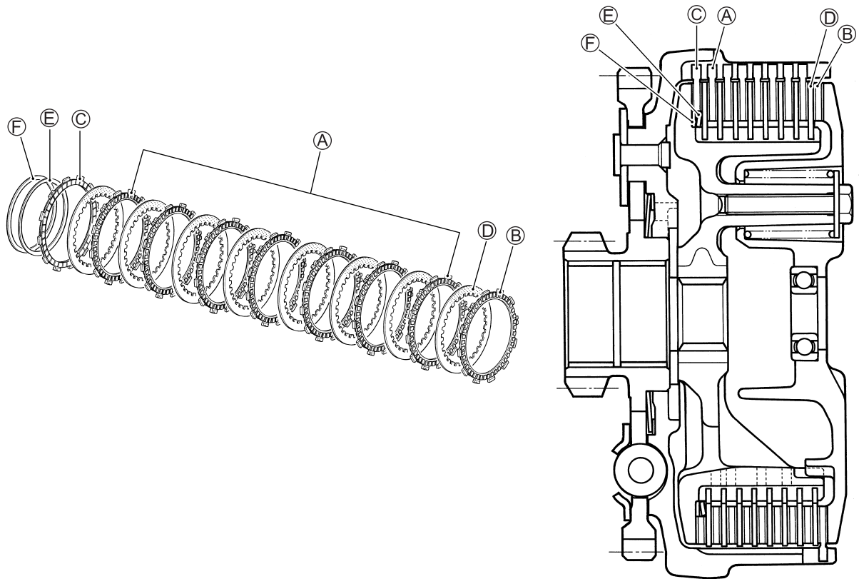
Ⓐ DISCO CONDUCTOR DE EMBRAGUE N.º 1 21441-29F00 (7 piezas)
