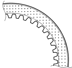
Ⓓ DISCO CONDUCTOR DE EMBRAGUE 21451-44D00
