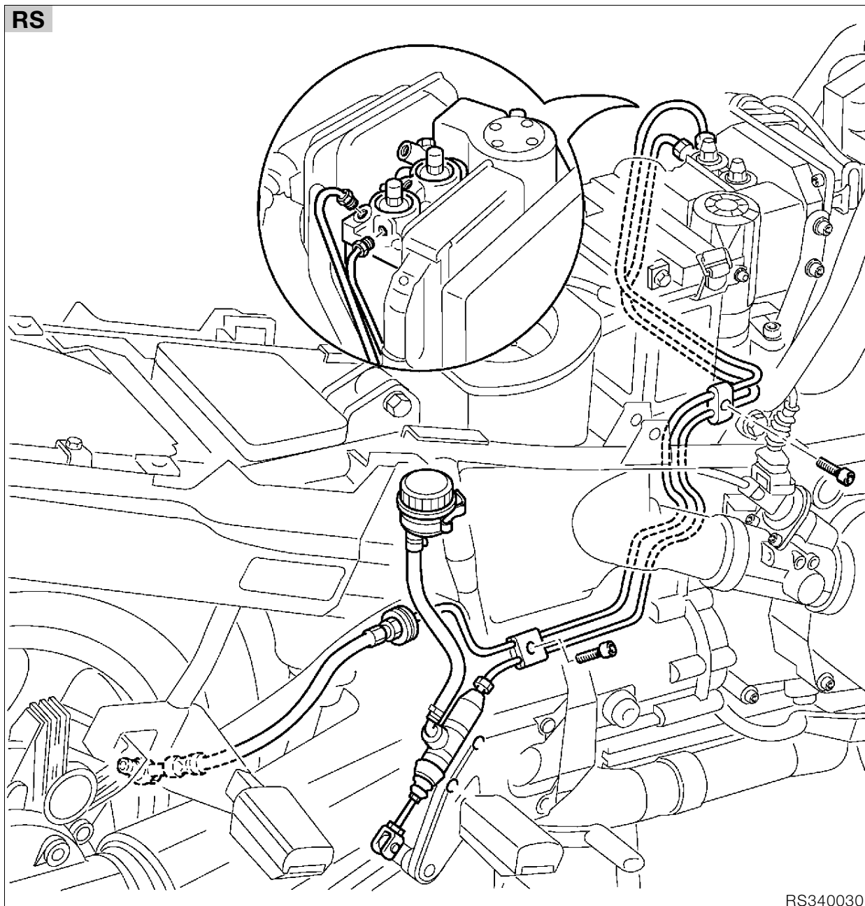
Desmontar y montar el conducto del líquido de frenos del ABS trasero
