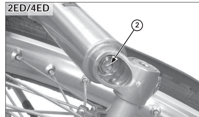
(2) REGULADOR DE COMPRESIÓN
