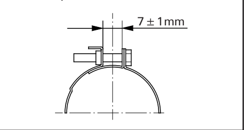
Banda aislante (lateral del cuerpo del acelerador):
