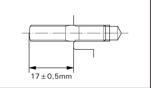
Espárrago del tubo de escape:
