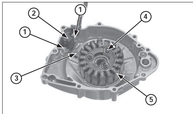
(1) tornillos (2) generador de impulsos de encendido (3) guía de cable (4) tornillos allen (5) estator
