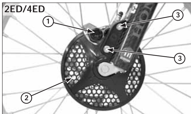
(1) PINZA DEL FRENO (2) TAPA DEL DISCO (3) TORNILLOS
