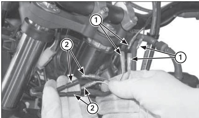
(1) CONECTORES INTERRUPTOR PARADA DEL MOTOR (2) CONECTORES INTERRUPTOR CABALLETE LATERAL
