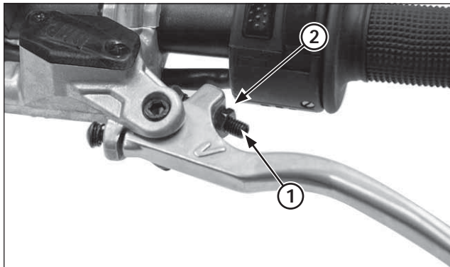
(1) REGULADOR (2) CONTRATUERCA
