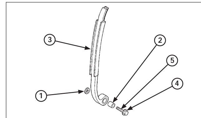
(1) ARANDELA (2) CASQUILLO DEL PIVOTE (3) TENSOR DE LA CADENA DE DISTRIBUCIÓN (4) TORNILLO DEL PIVOTE (5) APLIQUE AGENTE DE BLOQUEO
