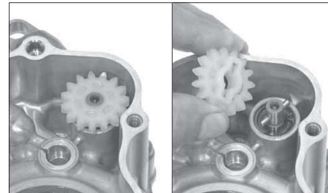
(1) ENGRANAJE CONDUCIDO (2) PASADOR DE ARRASTRE
