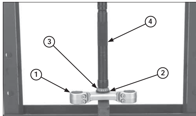
(1) TIJA DE DIRECCIÓN (2) GUARDAPOLVO (3) COJINETE (4) BOTADOR DE LA TIJA DE DIRECCIÓN
