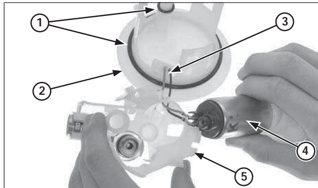
(1) JUNTAS TÓRICAS (2) BOMBA (3) CABLES DEL MOTOR (4) MOTOR (5) CUERPO
