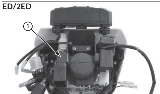
(1) RELÉ DEL MOTOR DEL VENTILADOR (ED/2ED)
