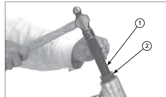
(1) BOTADOR (2) ACCESORIO
