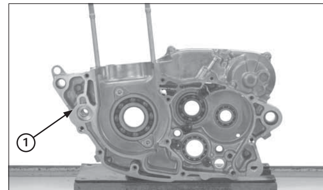
(1) CÁRTER DERECHO
