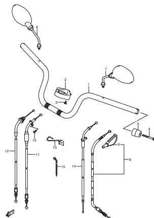
FIG.38 HANDLE BAR
