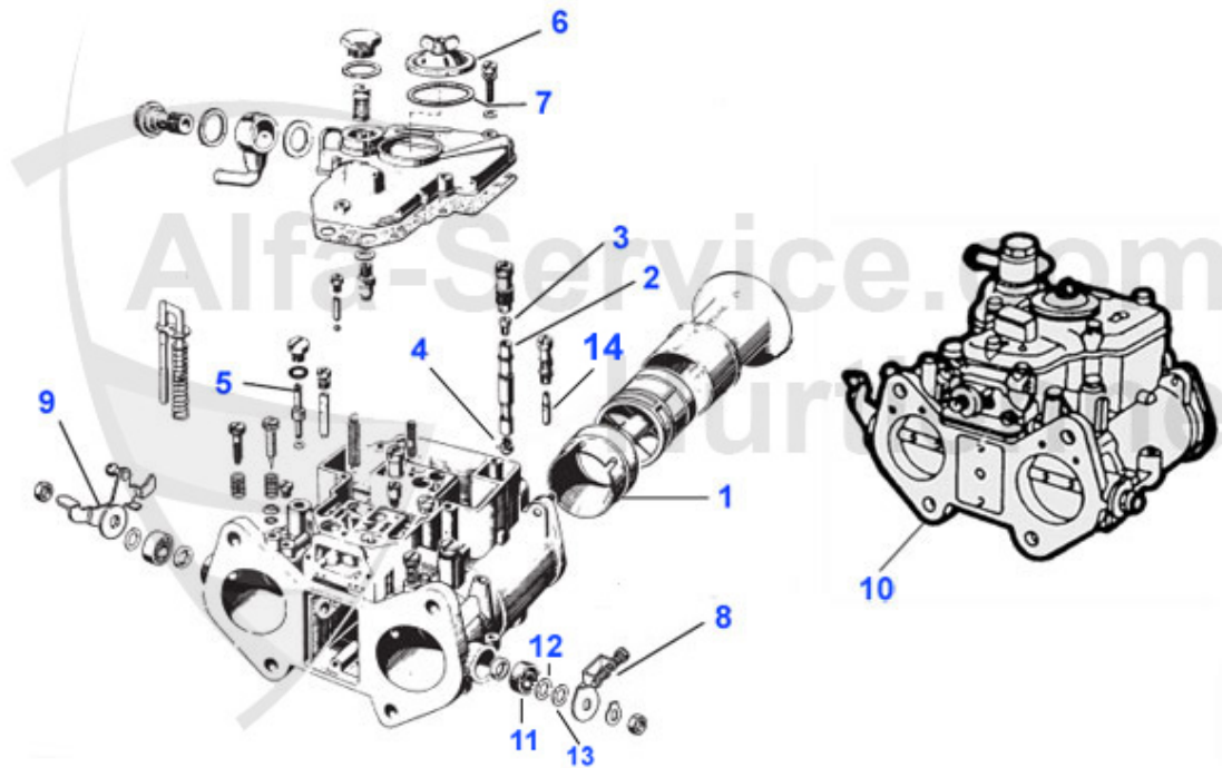
15 03 178 0 0 Schwimmer für Webervergaser Originalteil
