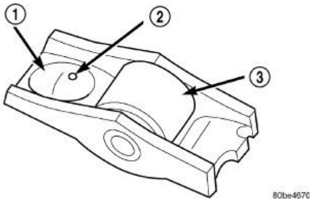
Fig. 272: Rocker Arm
