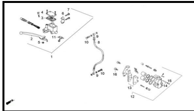
F-8 FRENO DELANTERO
