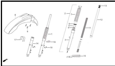
F-7 SUSPENSIÓN DELANTERA
