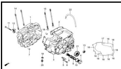
E-10 CARCAZAS CENTRALES
