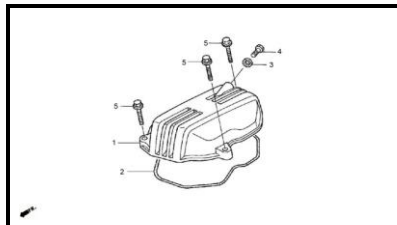
E-3 DISTRIBUCIÓN
