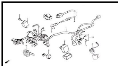
F-28 CHASIS
