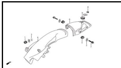
F-22 GUARDABARROS TRASERO
