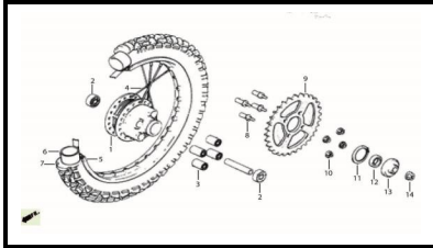
F-11 RUEDA TRASERA
