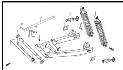
F-20 TIJERA / AMORTIGUADOR
