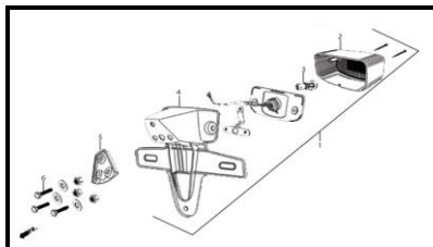
F-26 SISTEMA ELÉCTRICO 125
