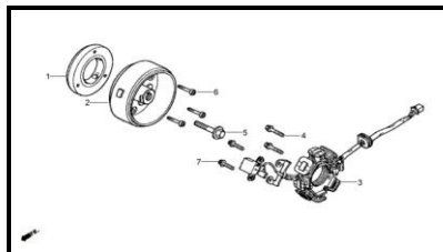
E-9 GENERADOR
