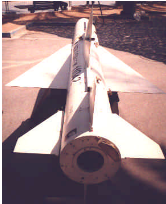
Misil R-530 equipado con motor cohete. Utiliza carburante sólido.
